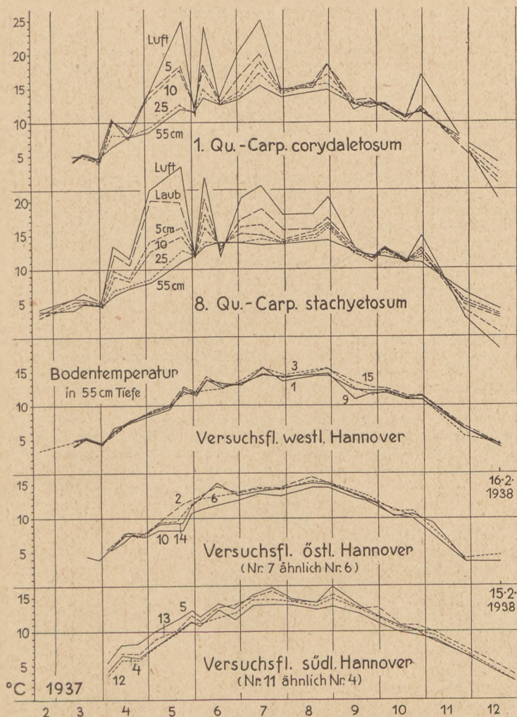
Abb. 12. Jahresgang der Luft- und Bodentemperaturen bei tiefem und hohem Grundwasserstand am Beispiel der Versuchsfächen Nr. 1 und 8, und Temperaturgang in 55 cm Bodentiefe für sämtliche Versuchsfächen.
