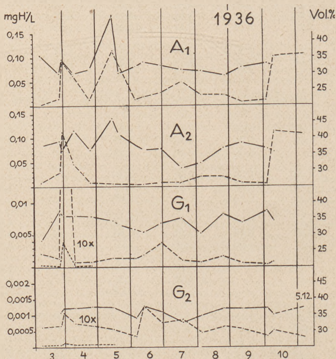
Abb. 35. Jahresgang der aktuellen Azidität und des Wassergehaltes in verschiedener Bodentiefe. — A. Querceto-Carpinetum stachyetosum Nr. 8, 1936, als Beispiel eines mäßig sauren Bodens. (Strichpunktirt = Wassergehalt in Vol. %, gestrichelt = Azidität in mg H + /L.)
