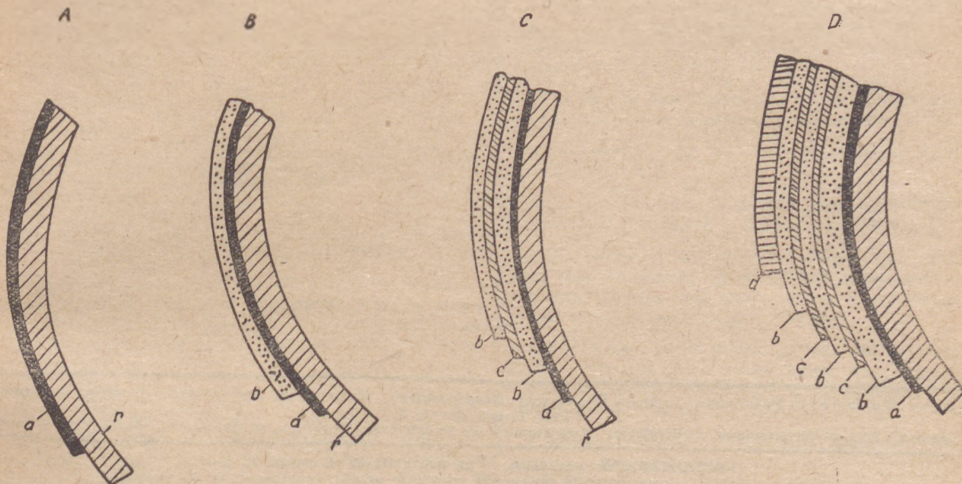
Różne rodzaje powłok, A - kryjąca, B - normalna, C - ciężka, D - bardzo ciężka r - rura, a - bitum, b - bitum z wypełniaczem, c - taśma nasyczona bitumem, d - plecionka słomiana
