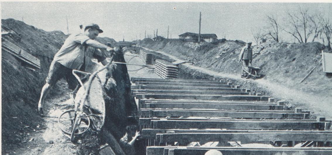
Главный канал длиной 4 км, по которому воды Росицы потекут на поля. Прокладка его идет к концу.
