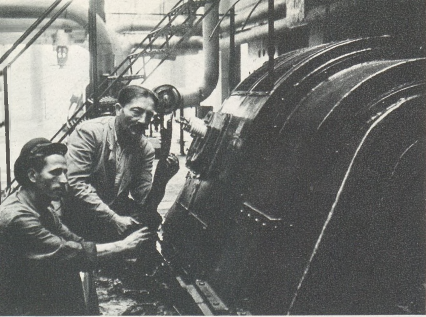
Руководитель электроремонтной бригады ТЭЦ „Республика“ Асен Захаринов и его помощник Кирилл Петров досрочно заканчивают ремонт.
