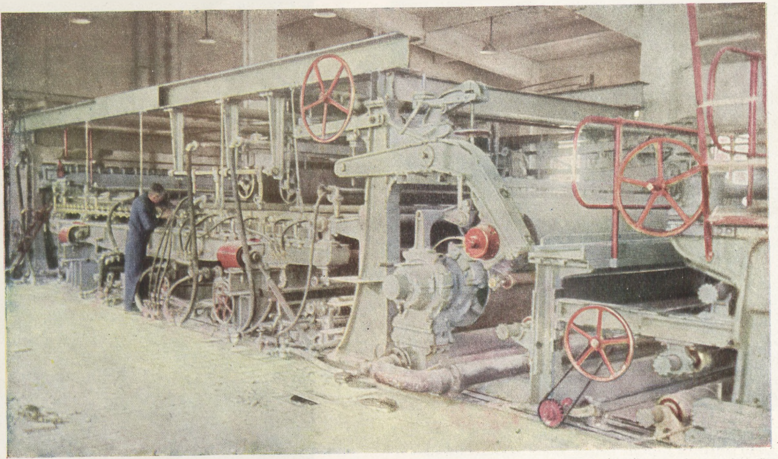
Монтаж главной машины для производства целлюлозы.
