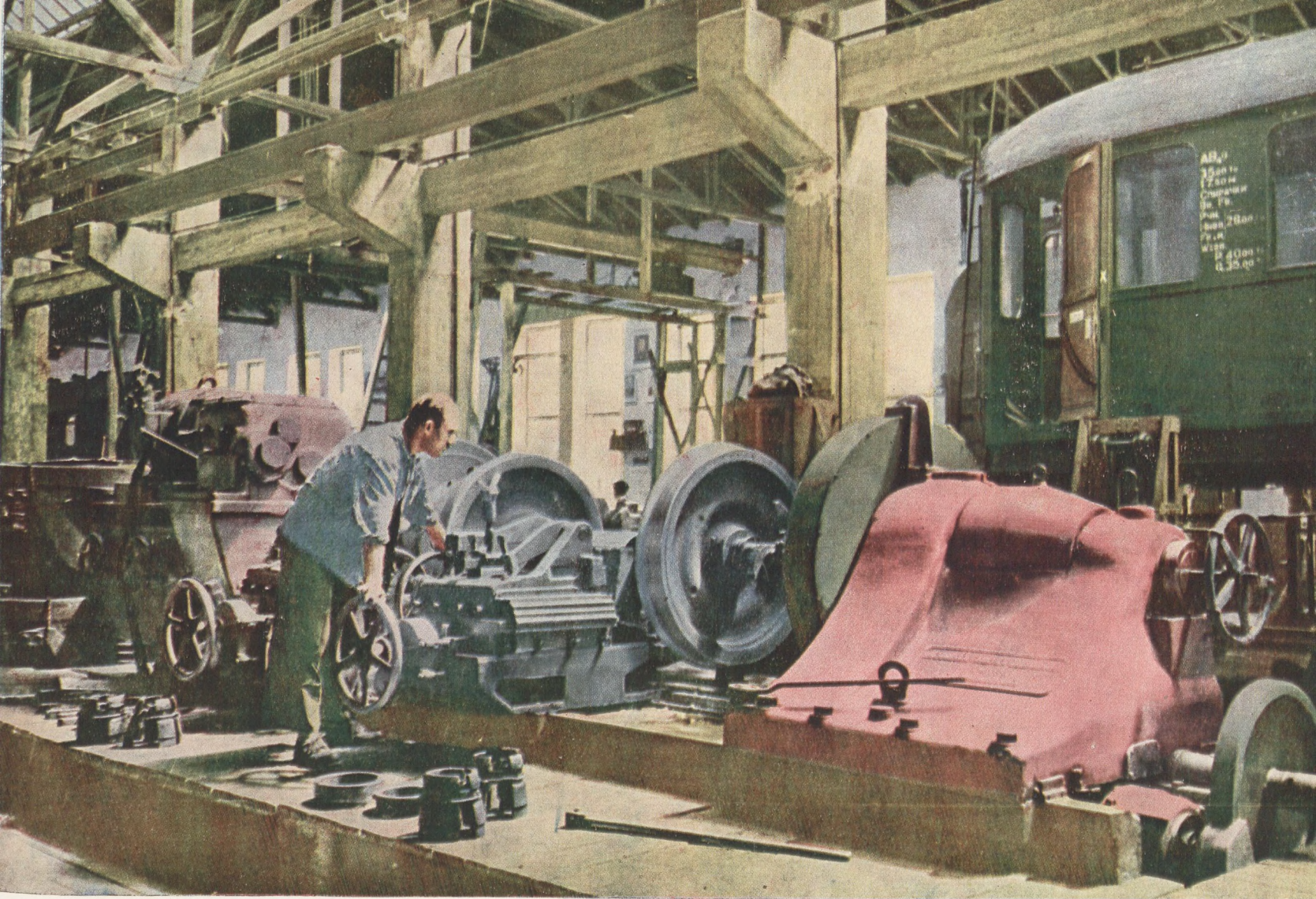
Мастер Цюню Кариев из демонтажного цеха за работой. Он один из первых в выполнении производственного плана.
