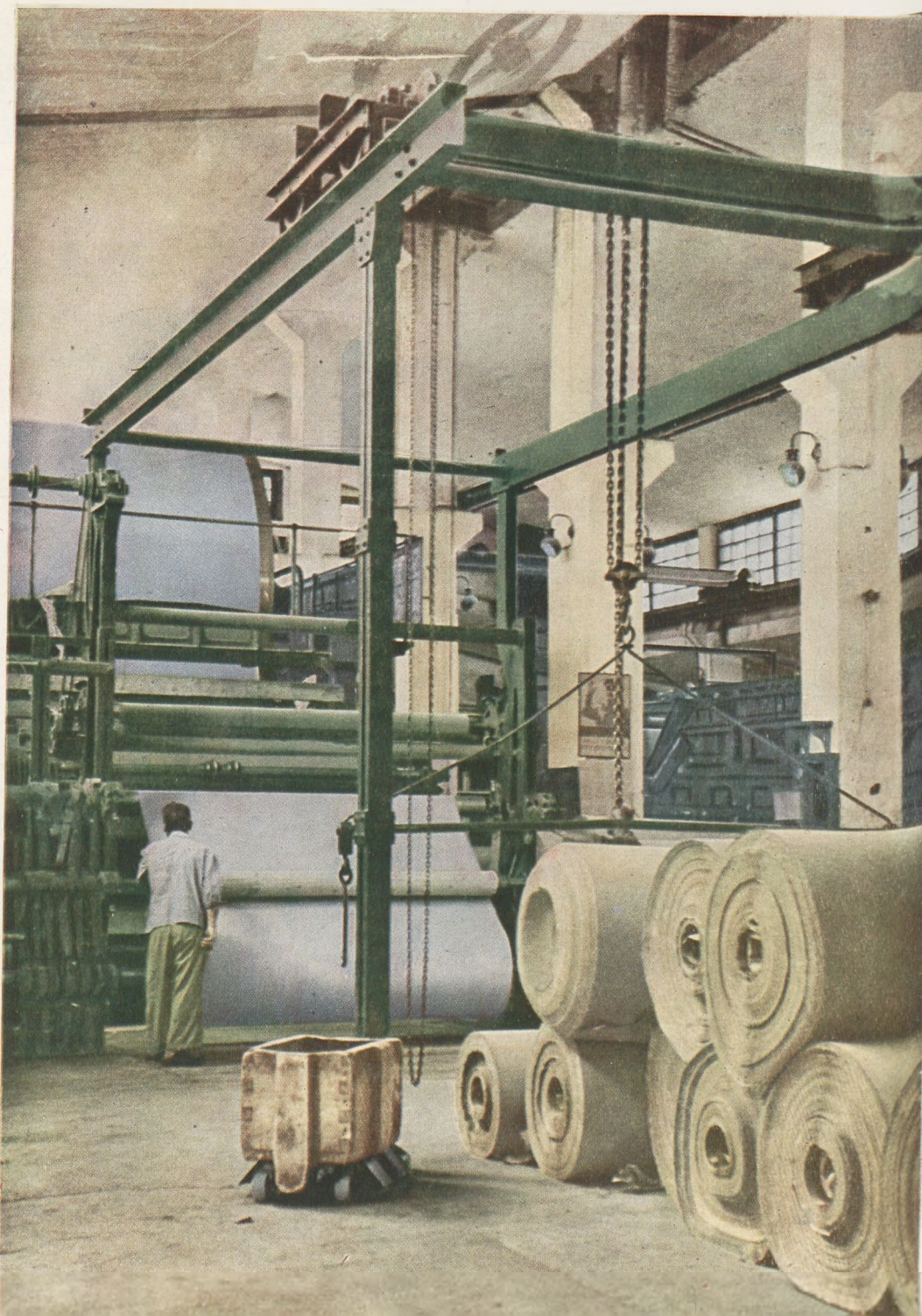
Машинный цех завода отличается высококачественным производством оберточной бумаги. На снимке: вторая машина.
