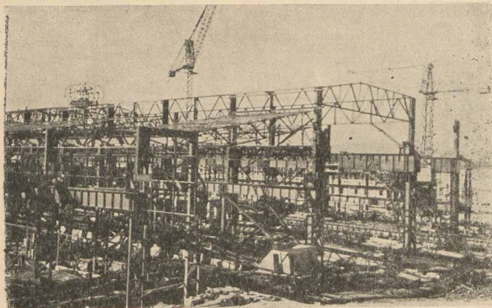
Мартеновский цех металлургического завода.
