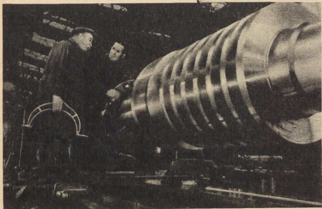
Obręcz jednego z cylindrów turbiny. Pracują przy niej ślusarze, Chochlaczew i Sugoniajew.
