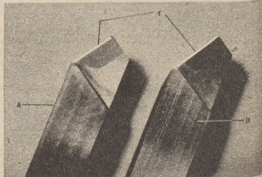
Noże, używane do skrawania metali. Ciemne miejsca przy górnych krawędziach — to ostrza z twardych spieków.
