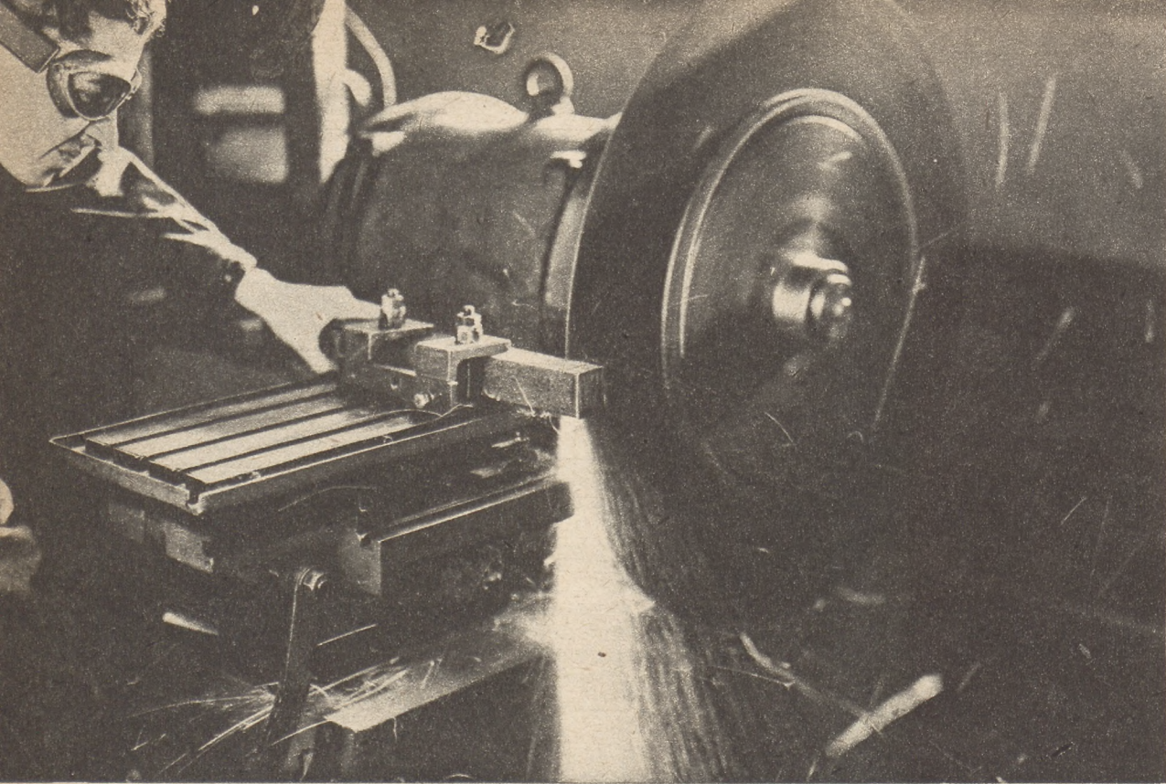
Wielka, nowoczesna piła cierna tnie metal z szybkością 450 km/godz. Przy takiej metodzie obróbki
