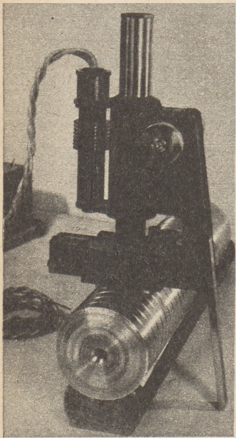
Przyrząd do mierzenia gładkości metalu, wynaleziony przez prof. Biernawskiego. Przyrząd pokazuje jakość obróbki...
