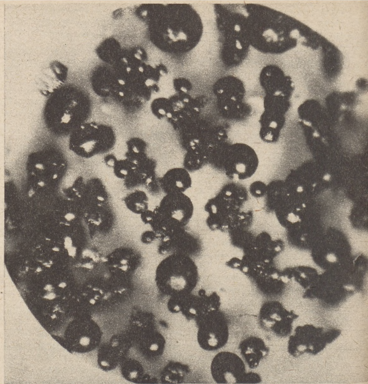
Wióry, które powstają przy cięciu piłą cierną w wysokiej temperaturze, widzimy pod mikroskopem jako kuleczki.
