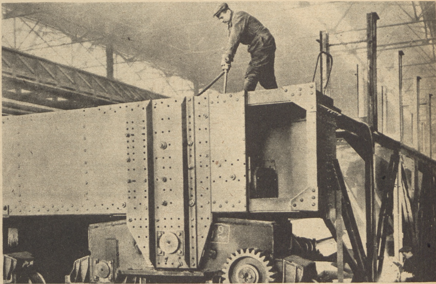
Montaż wielkiej suwnicy o nośności 300 ton. Przy produkcji suwnic racjonalizatorzy Nowo-Kramatorska zastosowali nową metodę spawania wielkich bloków metalowych, co umożliwiło skrócenie czasu trwania produkcji 350-tonowych suwnic hutniczych do połowy.
