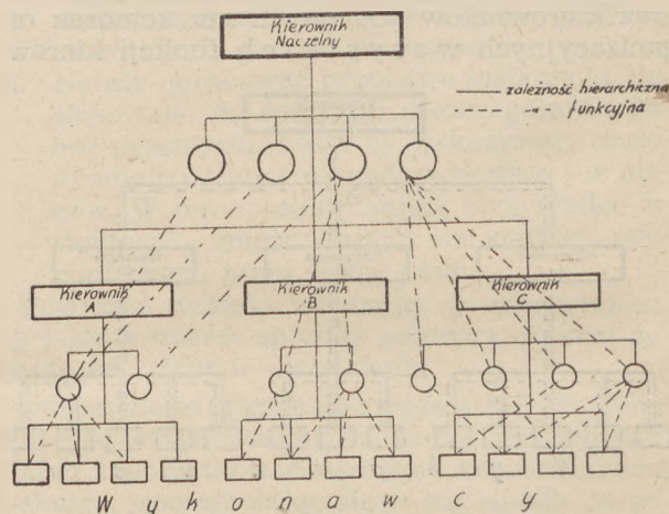
Rys. 3. System sztabowy
