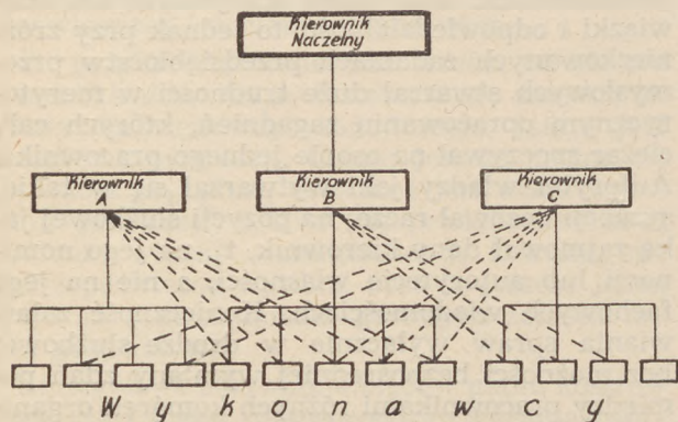
Rys. 2. System funkcjonalny
