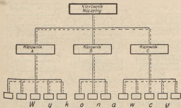
Rys. 1. System liniowy
