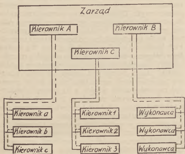
Rys. 4. System kolegialny
