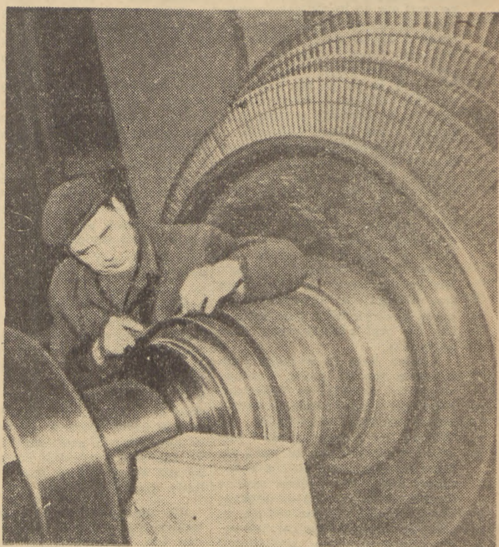
W budującej się elektrowni Jaworzno I trwa praca nad uruchomieniem pierwszego turbogeneratora. Na zdjęciu: monter Feliks Sarna przy montażu wirnika. Foto CAE — Wdowski
