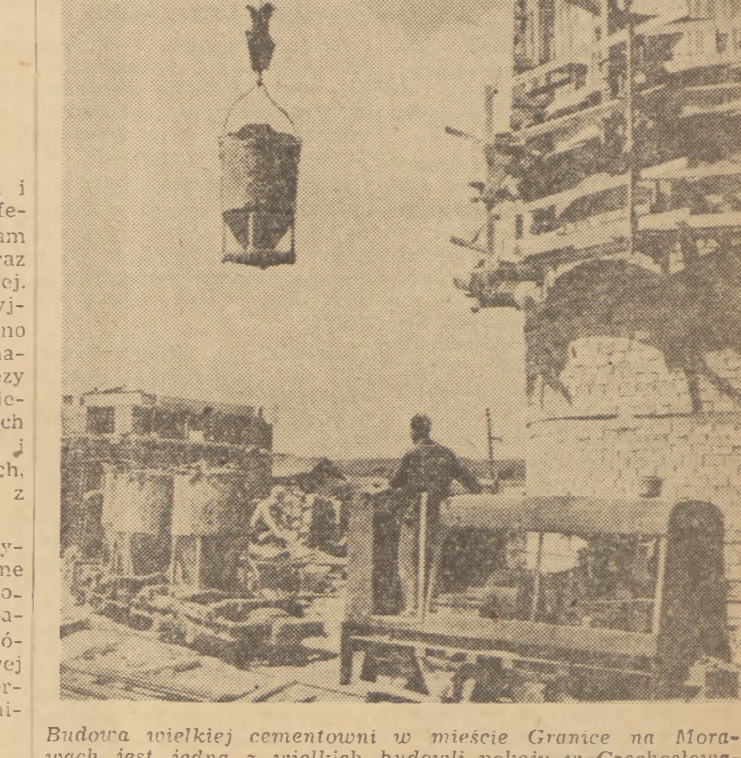
Budowa wielkiej cementowni w mieście Granice na Morawach. Jest jedną z wielkich budowli pokoju w Czechosłowacji. Na zdjęciu: prace przy budowie cementowni w Granicach. Foto CAP
