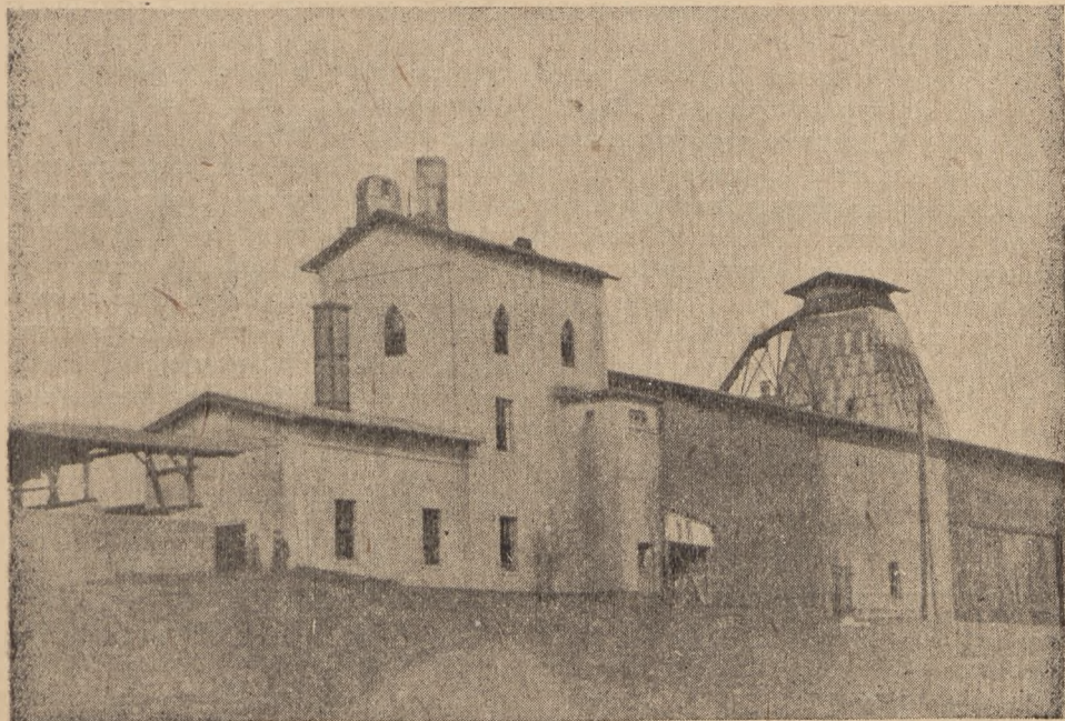
Fot. B. Suszarnia typu Rema-Rosin (pneumatyczna) (wygląd zewnętrzny budynku)
