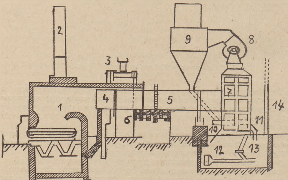
Rys. 4. Suszarnia bębnowa
