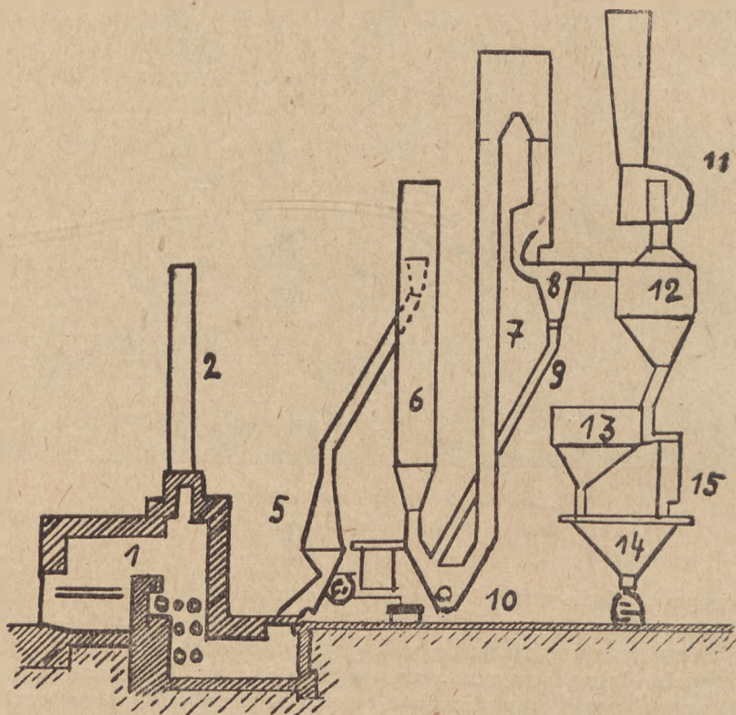
Rys. 5. Suszarnia pneumatyczna
