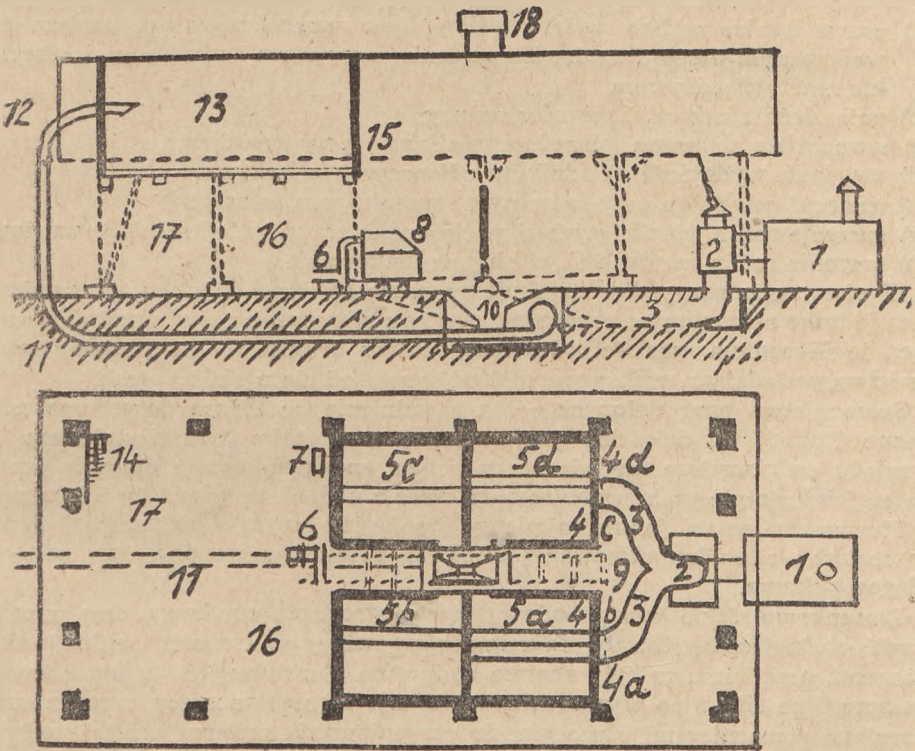
Rys. 1 i 2. Przekrój podłużny i poprzeczny suszarni sitowo-podłogowej
