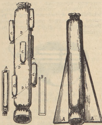
Rys. 5. Rakietą-matką holującą szeregiem mniejszych
