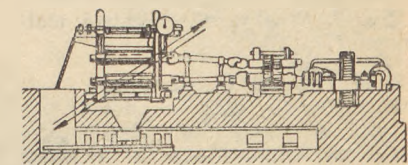
Rys. 5. Walcarka blach napędzana za pomocą maszyny parowej
