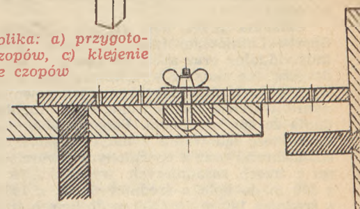
Rys. 8. Połączenie wsporników z poprzeczkami
