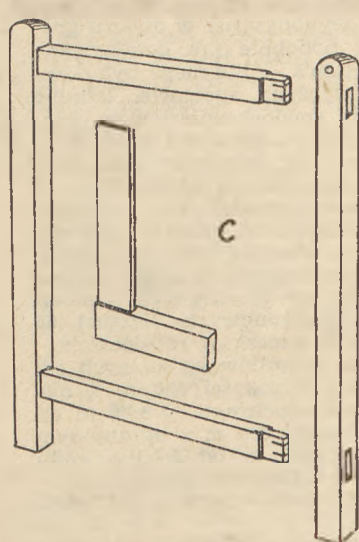
Rys. 5. Sklejanie elementów stolika: a) przygotowanie kliników, b) narzynanie czopów, c) klejenie i sprawdzanie kątów, d) klinowanie czopów
