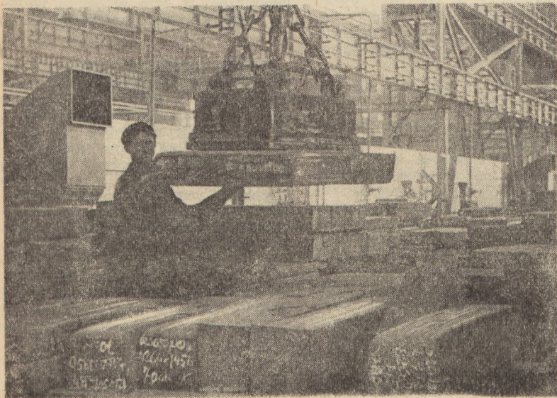
Rys. 16. Chwytnik elektromagnetyczny suwnicy wykończalni
