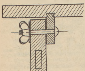
Rys. 7. Połączenie płyty stolika z nóżkami
