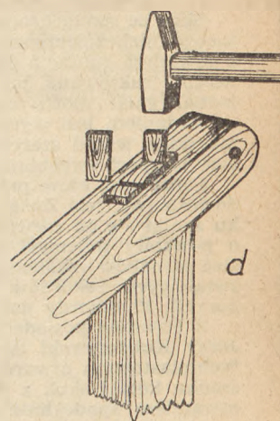
Rys. 3. Wyznaczanie i piłowanie czopów w listwach
