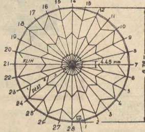
Czasza spadochronu. Rzut poziomy — w środku widoczny „kominek”
