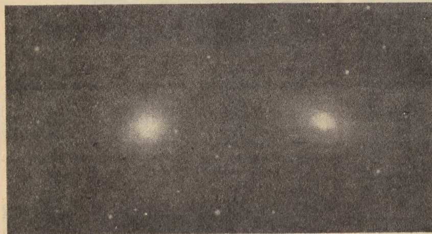
Rys. 2. Dwie galaktyki we Lwie, które właśnie zderzają się ze sobą.
