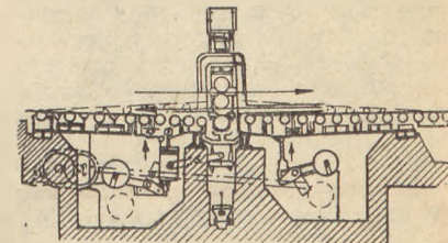
Rys. 6. Walcarka trio (3 walce) z samotokami wahadłowymi
