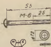
Rys. 4. Przygotowanie wsporników
