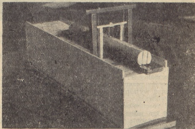
Obracając korbą (od strony niewidocznej na fotografii), wprawia się w ruch piły tego modelu traka tartaczego i jednocześnie zębate kółko przesuwające pień ku przodowi. Ten ciekawy eksponat wykonali członkowie Kółka Młodych Techników przy Szkole Podstawowej nr 8 w Przemyśle
