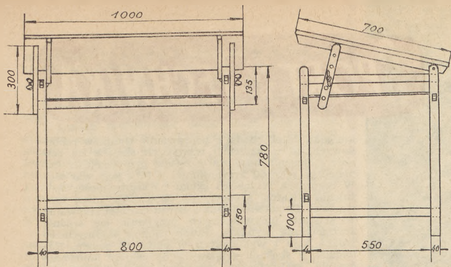
Rys. 1. Ogólny widok stolika
