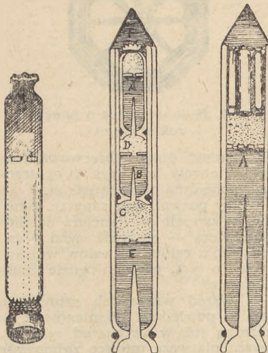
Rys. 2. Rakietą z łuską papierową
