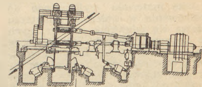
Rys. 7. Zgniatacz o 2 walcach poziomych napędzany silnikiem elektrycznym
