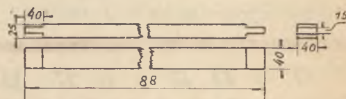
Rys. 3. Wyznaczanie i piłowanie czopów w listwach
