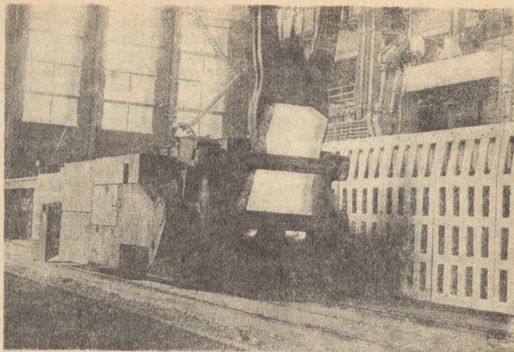
Rys. 10. Elektryczny wózek-wywrotka
