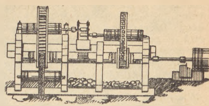
Rys. 3. Walcarka blachy napędzana za pomocą koła wodnego. Klatka, wały, koła zębate wykonane z drewna
