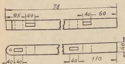
Rys. 2. Wyznaczanie i dłutowanie otworów w słupkach
