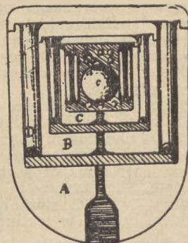
Rys. 10. Złożony pocisk rakietowy
