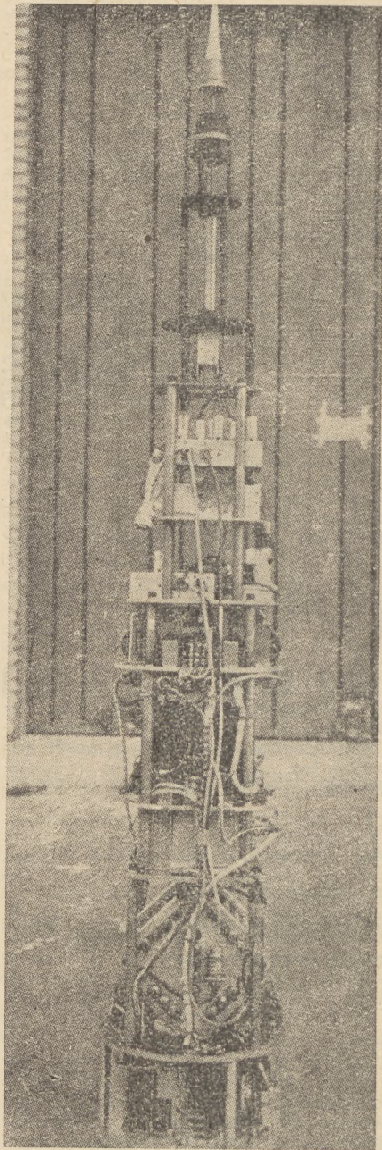
Rys. 3. Aparatura „Aerobee” przeznaczona do badania promieni kosmicznych
