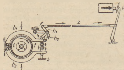
Rys. 12. Dźwignia hamulcowa samochodu
