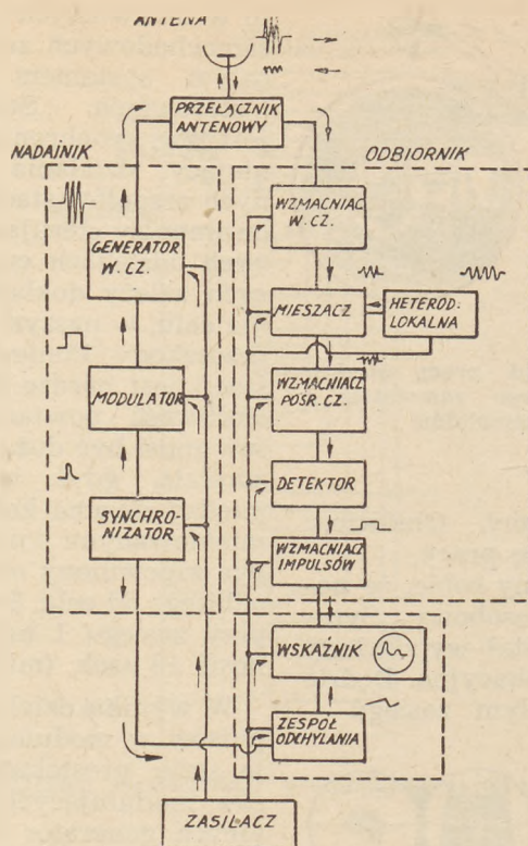
Rys. 10. Schemat blokowy stacji radiolokacyjnej
