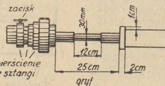
Hantle rozkładane do rozwijania siły mięśni rąk
