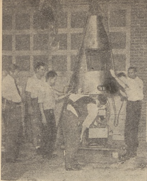
Rys. 4. Montowanie w dziobie „Aerobee” robotów obserwujących
