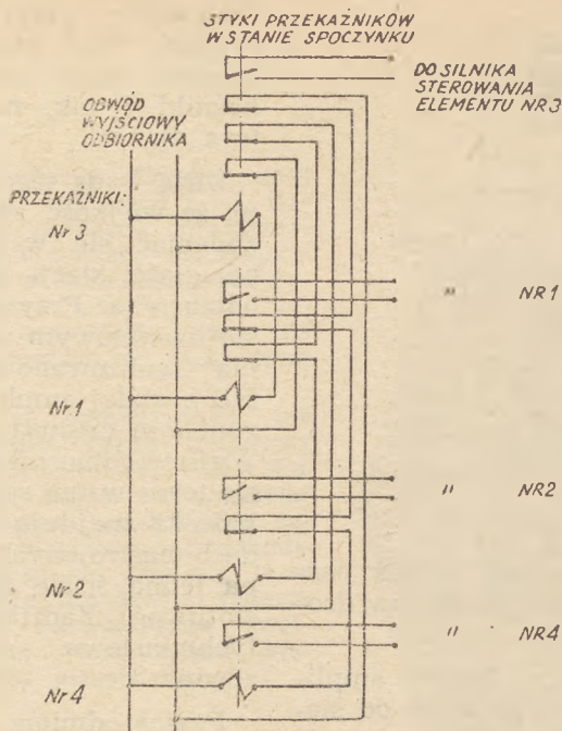
Rys. 4. Układ sterowania z przekaźnikami na różne amplitudy
