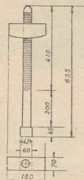
Rys. 3. Śruby drewniane
