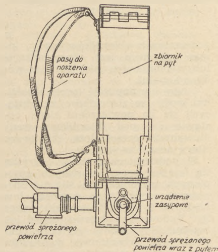
Rys. 4. Aparat do opylania wyrobisk
