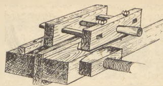
Rys. 13. Przystosowanie prasy do struga
