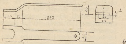
Rys. 8. a) klucz do nakrętek drewnianych, b) klucz do nakrętek metalowych
