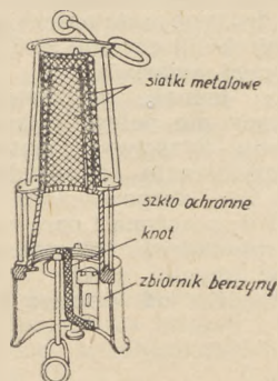
Rys. 1. Benzynowa lampa bezpieczeństwa
