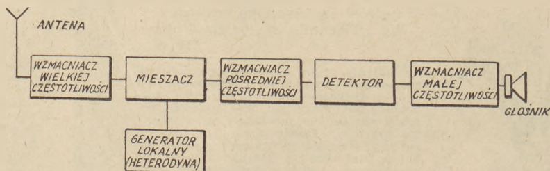
Rys. 1. Schemat blokowy odbiornika radiowego (superheterodynowego)
