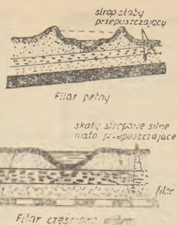
Rys. 7. Filary ochronne pod zbiornikami wodnymi na powierzchni ziemi
