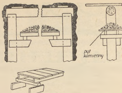
Rys. 3. Zapora z pyłu kamiennego
