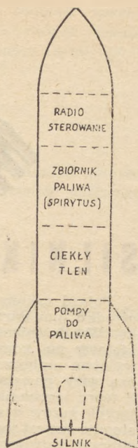
Schemat rakiety V-2
