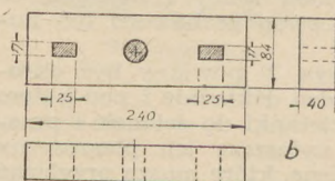
Rys. 9. Sposób unieruchamiania prasy na stole
