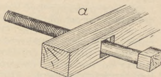
Rys. 5. Zamocowanie śrub w belce: a) drewnianej, b) metalowej
