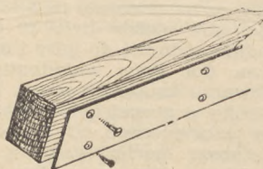
Rys. 6. Zabezpieczenie boku belki blachą
