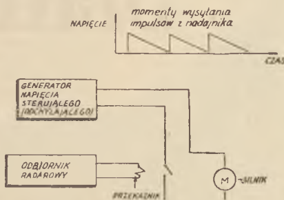
Rys. 14. Schemat blokowy uruchamiania hamulców
