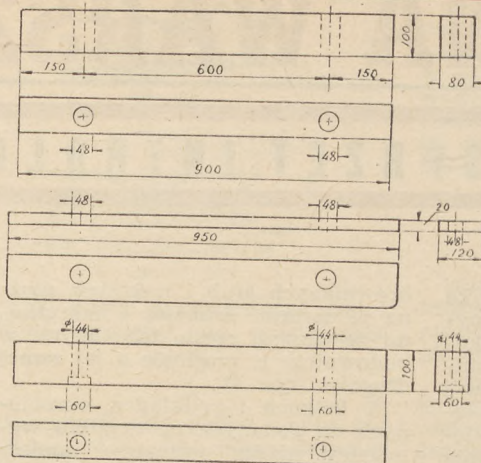
Rys. 2. Belki i podkładka
