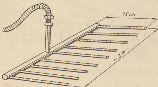
Rys. 3. Urządzenie do parowania ziemi
