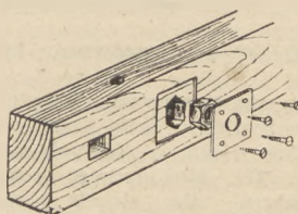
Rys. 14. Osadzenie nakrętki metalowej w klocku (b)
