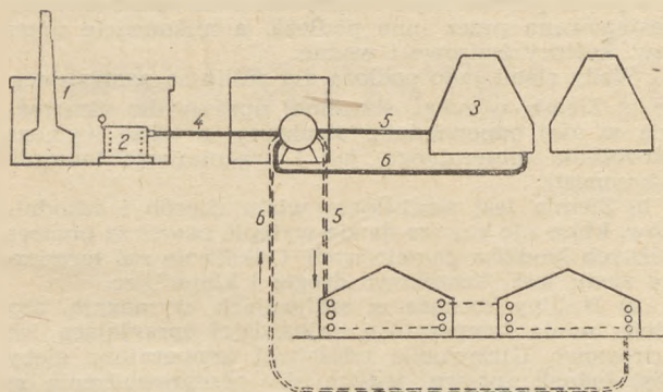
Rys. 1. Schemat wykorzystywania ciepła odpadkowego z elektrowni do ogrzewania szklarni zamiast bezproduktywnego chłodzenia pary w chłodnicach kominowych: 1 — elektrownia, 2 — kotłownia, 3 — chłodnice kominowe, 4 — para o wysokim ciśnieniu, 5 — para o niskim ciśnieniu, 6 — woda
