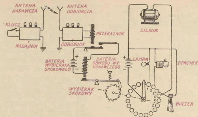
Rys. 2. Schemat najprostszego układu sterowania za pomocą radia
