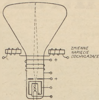
Rys. 13. Lampa obrazowa radaru
