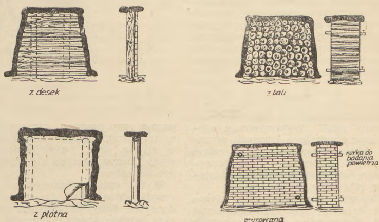
Rys. 5. Tamy ogniowe
