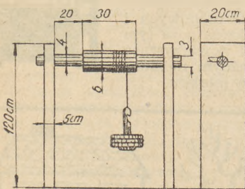
Kołowrót do ćwiczeń nadgarstka
