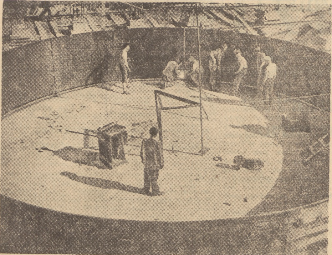
Złota „Mostostni” z Nowej Huty podjęła niedawno zobowiązanie przyspieszenia montażu płaszczy trzech nagrzewnic oraz Wielkiego Pieca nr 1 o 70 dni. Na zdjęciu: brгада тов. Дылонга przy spawaniu pierwszego pierścienia pancera Wielkiego Pieca nr 1. Foto — A. Nowosielski
