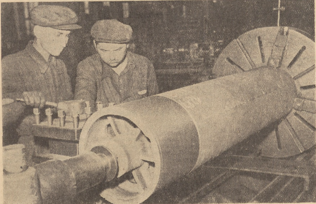
Przy użyciu zwykłego noża tokarskiego i przy dużym pośpiechu obróbka widocznego na zdjęciu wata trwała w Z.U.T. „Zgod” 22 godziny. Po zastosowaniu noża Kolesowa ta sama operacja trwa — 12 godzin. Foto A. Nowosielski
