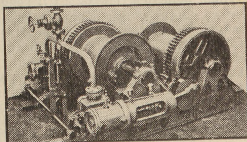
Parowa maszyna wydobywczą.
