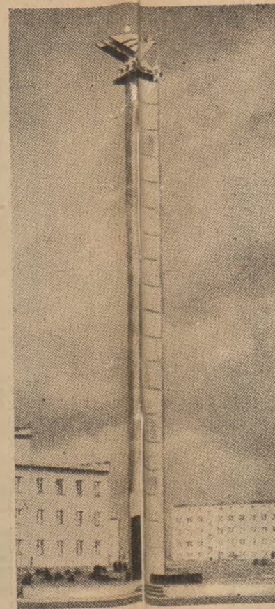
Obelisk ku czci Marszałka J. Piłsudskiego na Lotniku wg. projektu inż. Ochmańskiej-Mrówkowej.
