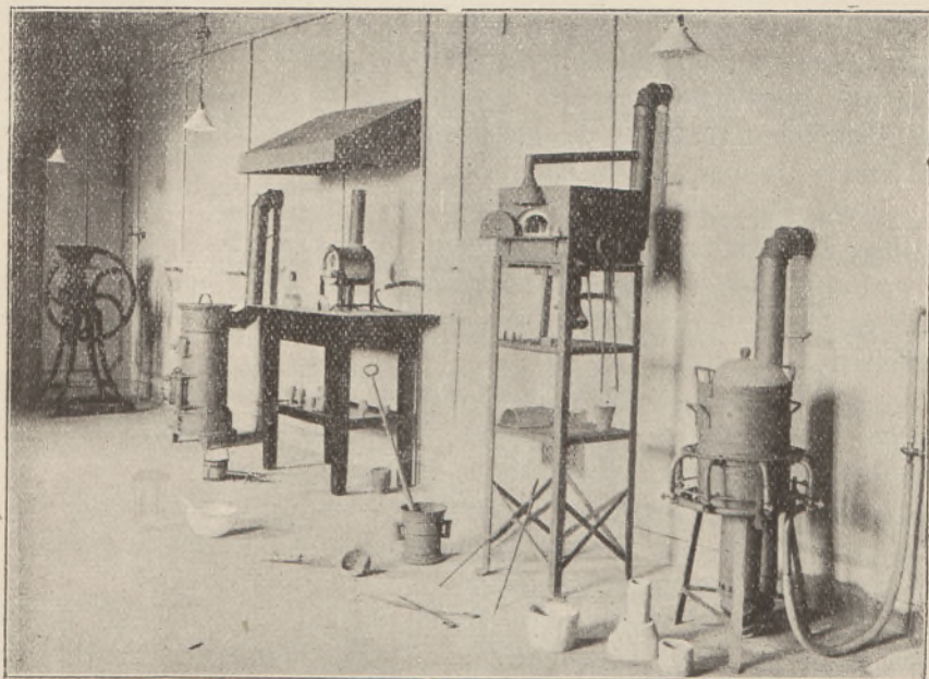
Mahlapparat.
