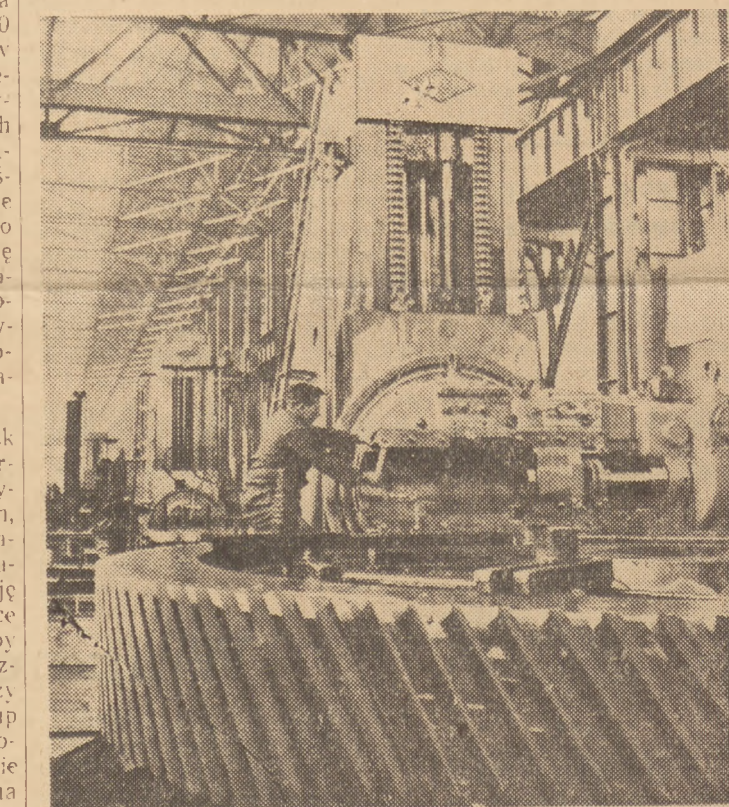
Nowokramatorskie Zakłady im. J. Stalina (Ukraińska SRR) produkują maszyny dla przemysłu ciężkiego. Na zdjęciu: obróbka olbrzymiego koła zębatego
