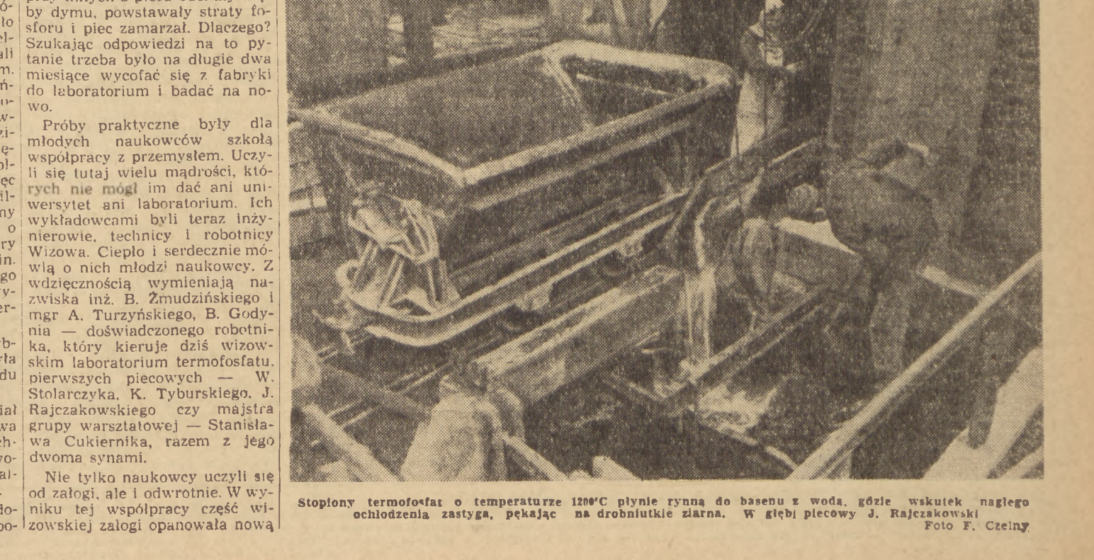
Stopiony termofosfat o temperaturze 1200°C płynie rynną do basenu z wodą, gdzie wskutek nagłego ochłodzenia zastyga, pękając na drobniutkie ziarna. W głębi piecowy J. Rajczakowski. Foto F. Czelny
