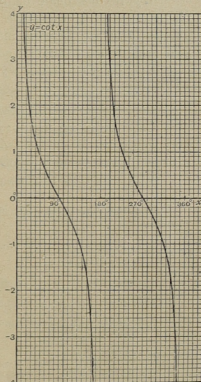
y = \cot x.
