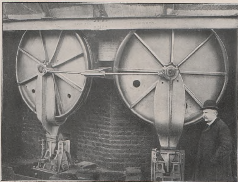
Die beiden Entlastungsrollen des großen Fernrohrs der Treptow-Sternwarte.
