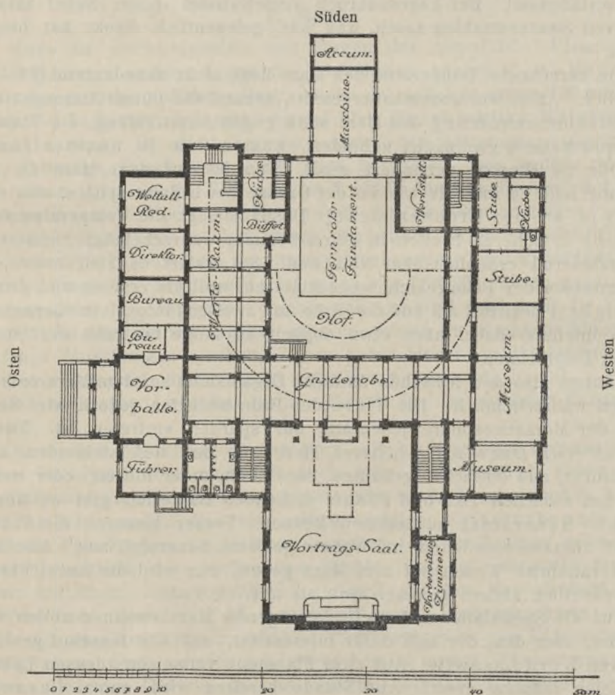
Grundriß des Neubaues der Treptow-Sternwarte.
