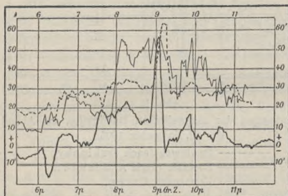
Abb. 2. Schwankungen der magnetischen Deklination am Abend des 15. November 1905. — Pawlowsk (nach Dubinsky). - - - Potsdam (nach A. Schmidt). ... Kew (nach Chree).
