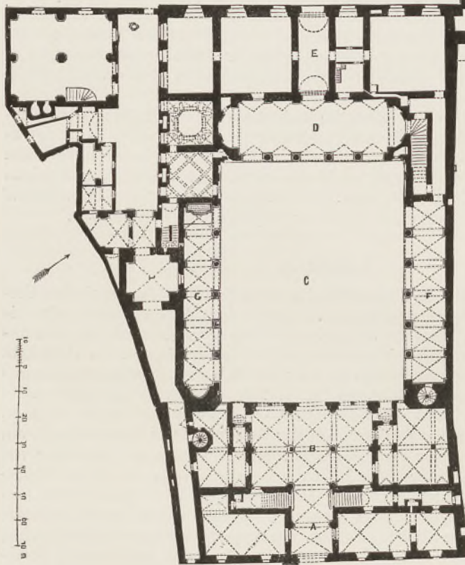
Abb. 2 Grundriß der Neuen Residenz zu Landshut
