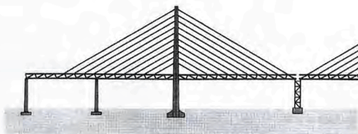
Schemat organizacji montażu mostu: najpierw wykonano monolityczne pylony, a następnie pływający żuraw „Łabędź” układał prefabrykowane elementy przęsła, które podwieszano do pylonów za pomocą kabli
