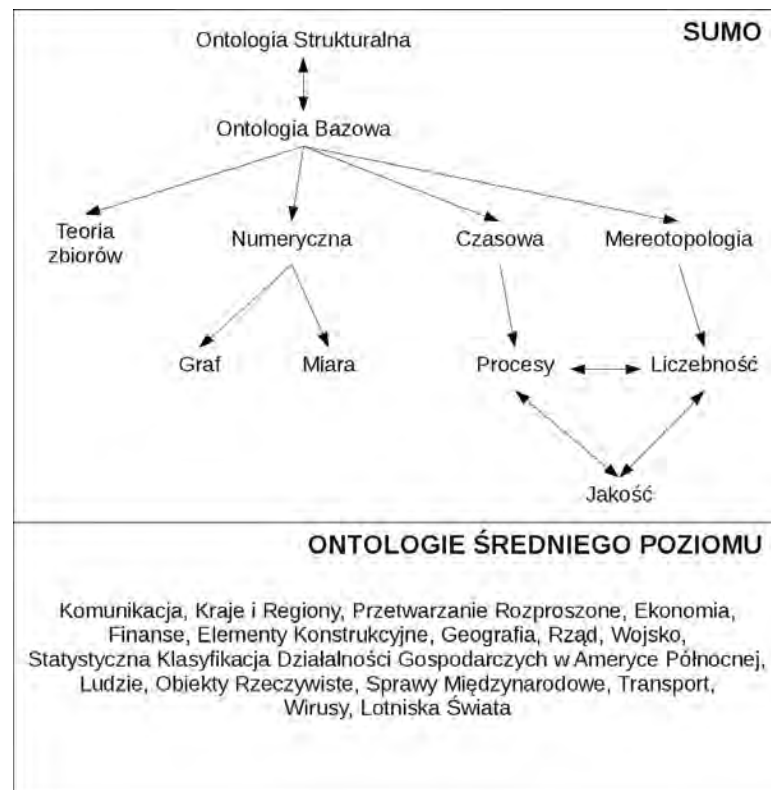
Rysunek 3.2: Wysokopoziomowa struktura ontologii SUMO i związanych z nią ontologii pochodnych [118]
