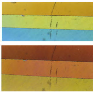
Fot. 7. Zdjęcie polaryzacji chromatycznej występującej w jednej, dwu i trzech warstwach celofanu nałożonych kolejno na siebie, dla dwu kątów skręcenia płaszczyzn przepuszczania między polaryzatorem a analizatorem
