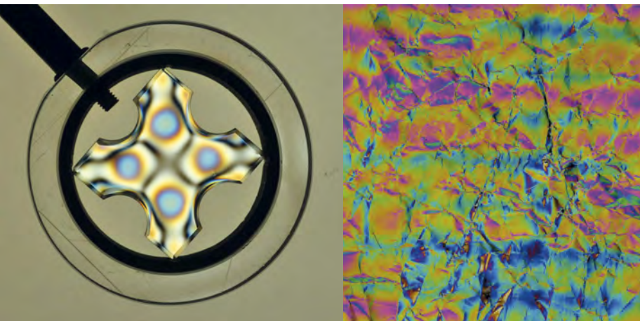
Fot. 4. Obraz rozkładu naprężeń w płytce szklanej. Isochromy są to obszary powierzchni o tej samej barwie. Odpowiadają im te same wartości naprężeń
