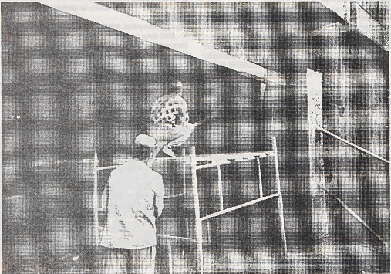
Wykonywanie prac renowacyjnych metodą torkretowania
