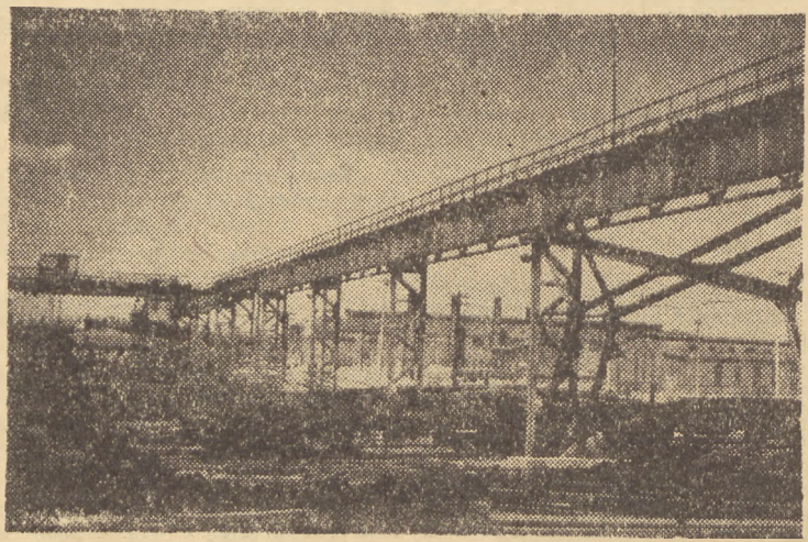
Z każdym dnem rośnie — duma całej Polski — Kombinat Metalurgiczny Nowa Huta. Na zdjęciu: Fragment transportera międzyhalowego (estakady), który służy do rozładowywania i dostarczania surowców do poszczególnych hal produkcyjnych Kombinatu. CAF. — fot. Tyński
