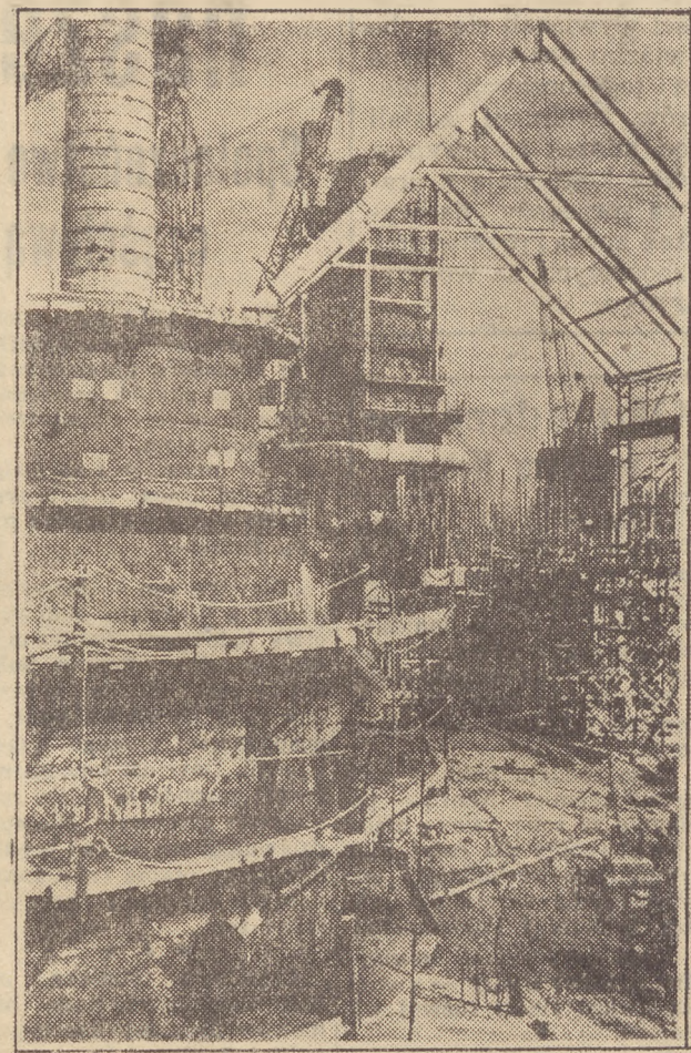
Rejon wielkich pieców w Nowej Hucie. Montaż pancernia i nagrzewanie wielkiego pieca nr 2.
