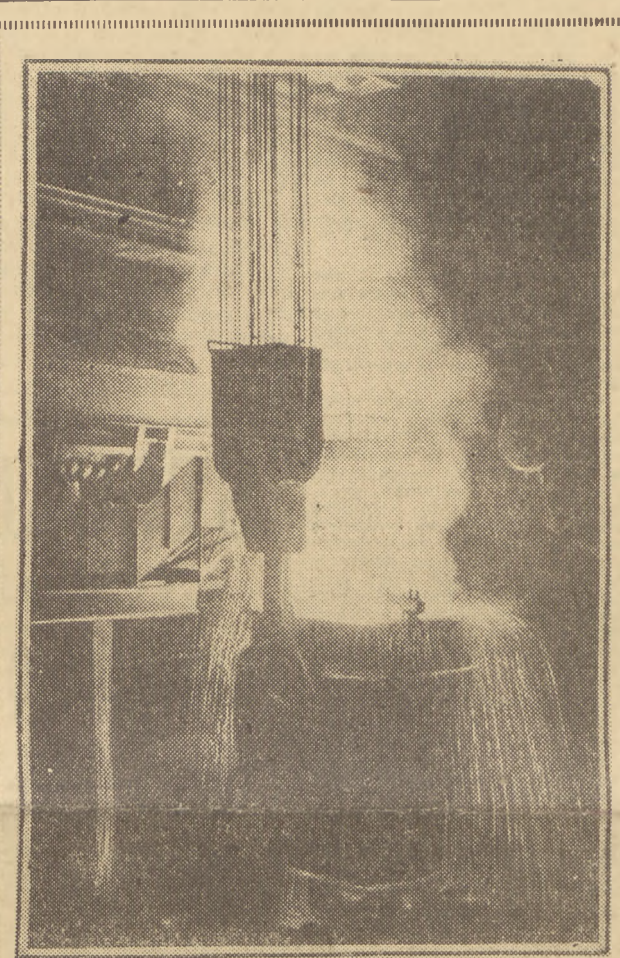
W dniu 4 lutego 1955 r. z pieca martenowskiego Nr 1 Huty im. Lenina popłynęła pierwsza stal. Na zdjęciu: Spust stali. Stal z napełnionej kadzi wlewana jest następnie do wlewniczek.
