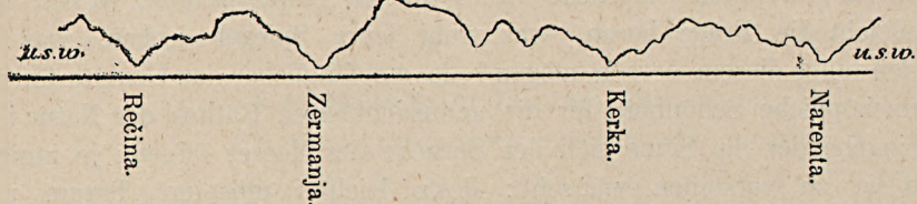
Ideales Längenprofil der Ostküste der Adria.
