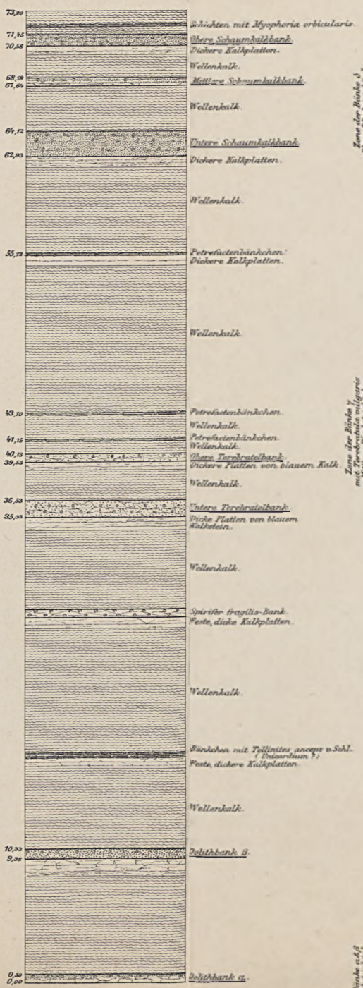
Fig. 2. Durchschnitt durch den Oberen Wellenkalk bei Meiningen.
