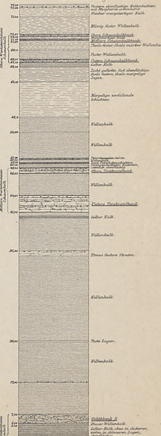
Fig. 1. Durchschnitt durch den Oberen Wellenkalk am linken Diemelufer zwischen Liebenau u. Osthelm unfern Warburg.
