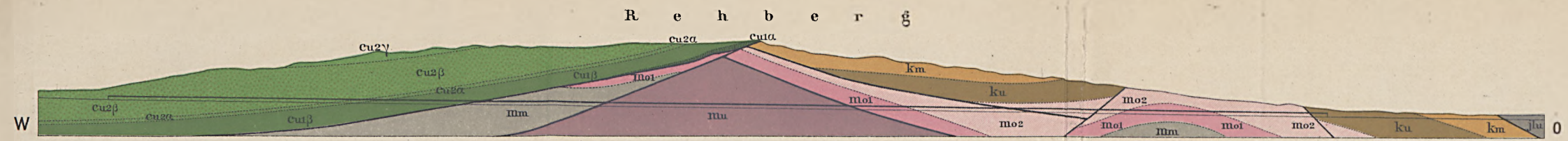
O-W Profil durch den grossen Tunnel von Altenbeken.
