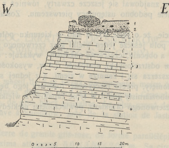
Fig. 30. Profil schematyczny wschodniej ściany kamieniołomu: a—głaz. 1. piaski dyluwjalne, 2. rumosz wapienny, 3. białe wapienie margliste, 4. wap. nerineowe (3—4 jura górna).
