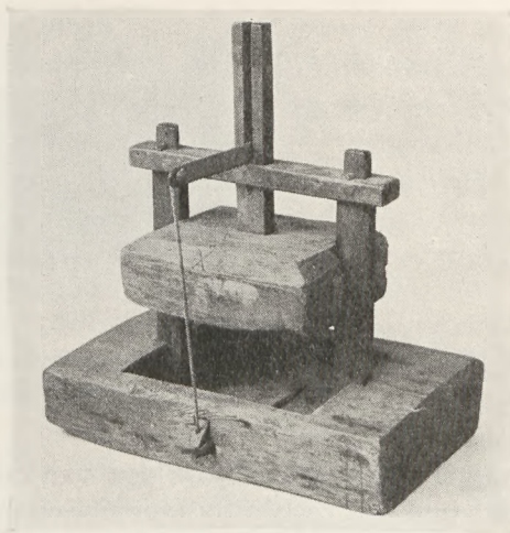
Fig. 9. Råttfälla med klumpkonstruktion. Näs socken, Dalarna. Nordiska museet.
