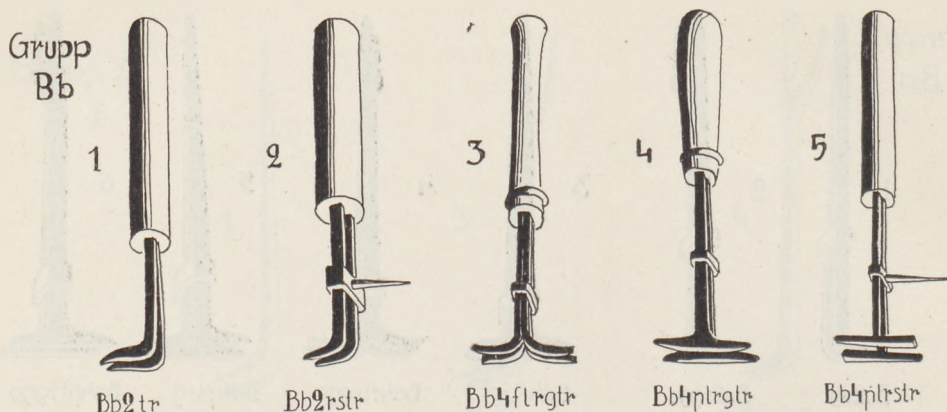
Fig. 3. Dragjärn med helkluven eller dubbel stjälk (typ Bb).
