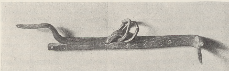
Fig. 28. Dragjörn med golvdrag och klingringar. Daterat 1750. Från Delsbo socken, Helsingland.
