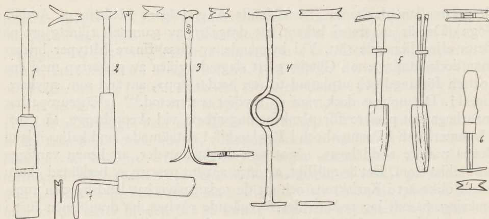
Fig. 14. Norske dragjærn. Norsk folkemuseum, Bygdö, Oslo. 1 från N. Helgeland, 2 från Gudbrandsdalen, 3 från Kongsvinger, 4 från Voss, 5 från Grimstad, 6 från Sogn, 7 från Kongsvinger. H. Vreim delin.
