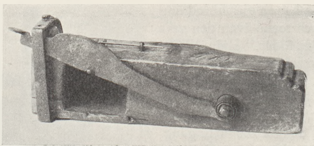
Fig. 10. Rättfälla med stålffjäder. Daterad 1704. Grängärde socken, Dalarna. Nordiska museet.
