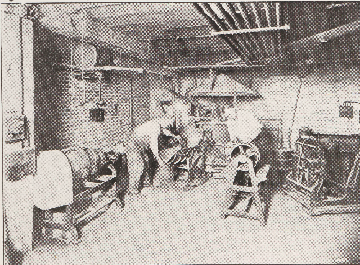
Styrotypia Dziennika Zjednoczenia, gdzie odlewa się płyty. Pod daszkiem widzimy kociół, w którym topi się metal. Na froncie dwie maszyny do obcinania płyt.
