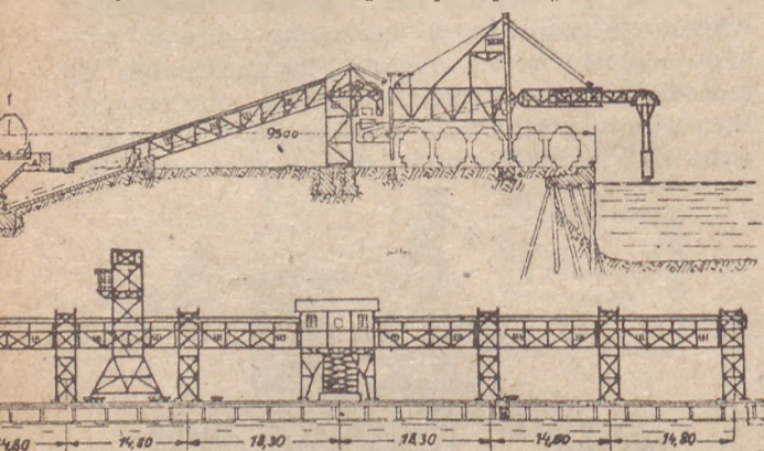
RYS. 10 Urządzenie taśmowe w Gdańsku
