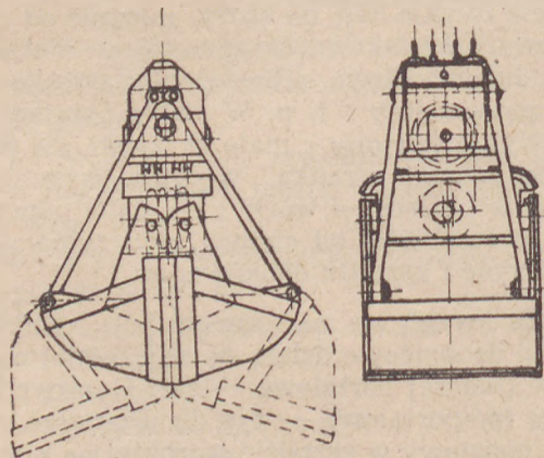
RYS. 4 Chwytnak
