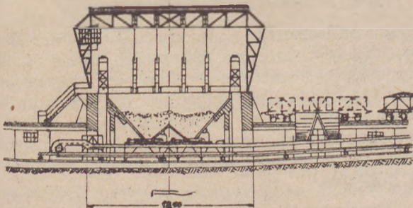
RYS. 7 Wywrotnica wagonowa. Widok z boku
