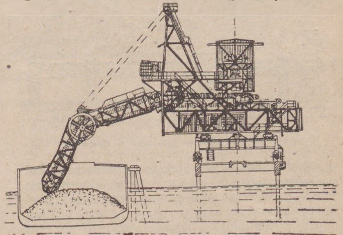
RYS. 9 Urządzenie taśmowe w Gdyni. Widok z przodu
