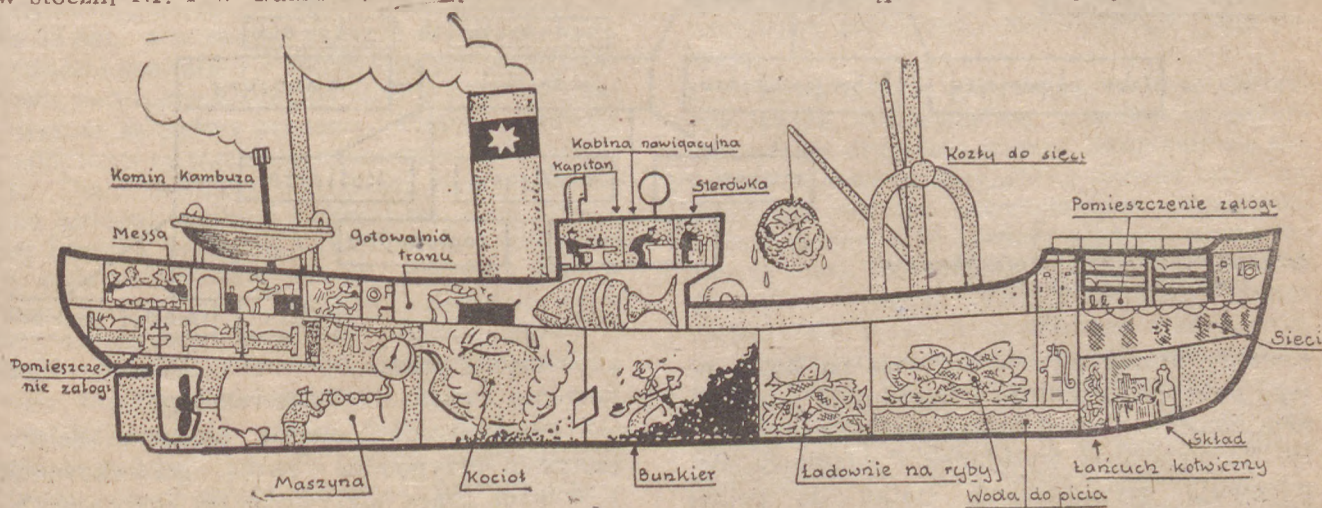
Pogłądowy przekrój trawlera rybackiego
