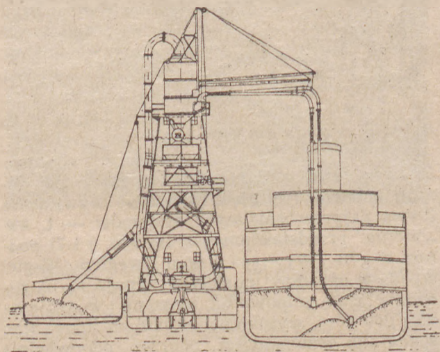
RYS. 11 Pływający elewator zbożowy
