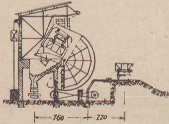
RYS. 6 Wywrotnica wagonowa Widok z przodu
