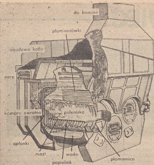
KOCIOŁ RUDOWĘGLOWCA
