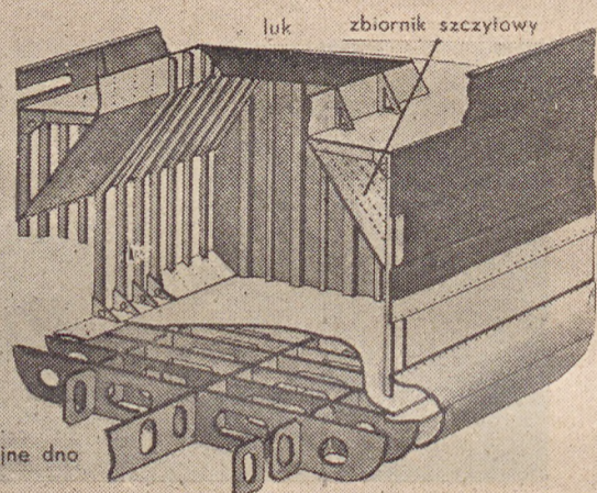
FRAGMENT ŁADOWNI RUDOWĘGLOWCA
