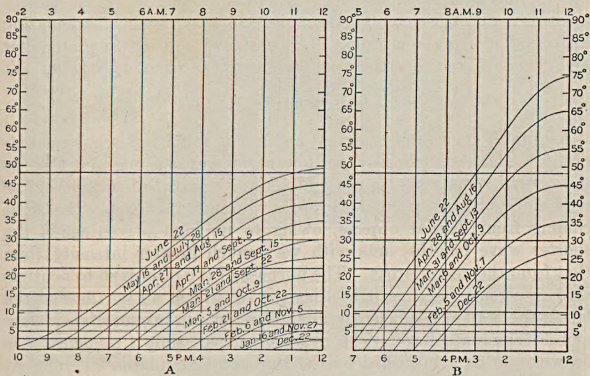
FIGURE 2.—Curves of sun's altitude. A, Latitude 39° N.; B, latitude 64° N.
