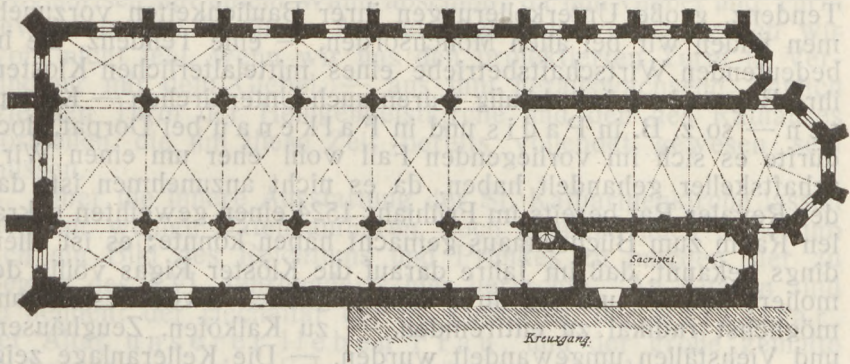
Abb. 29. Grundriss der Dominikanerkirche in Regensburg.
