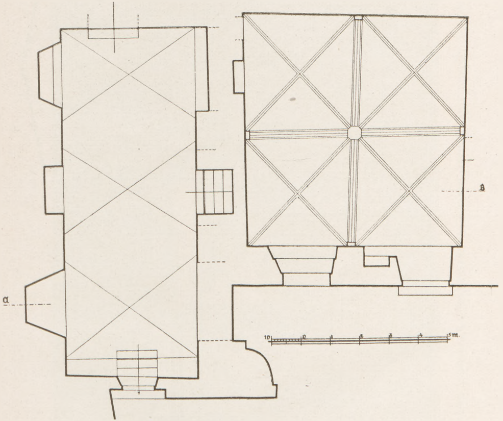
Abb. 13. Grundriss der Gervekammer und des Kapitelsaales.
