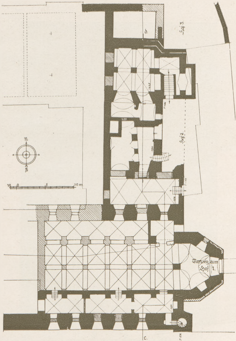
Abb. 8. Kellergrundriss.
