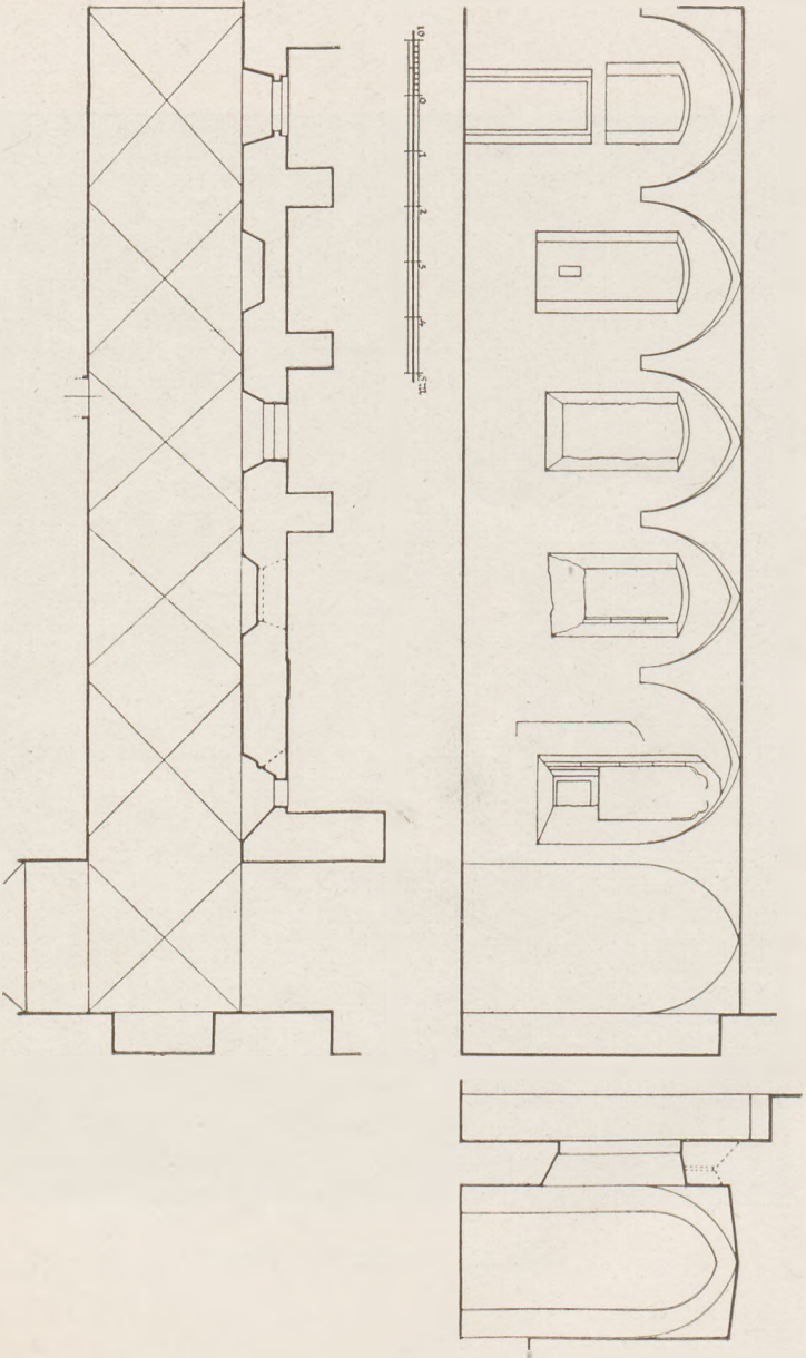
Abb. 16. Grundriss und Schnitt des Westreuzganges.
