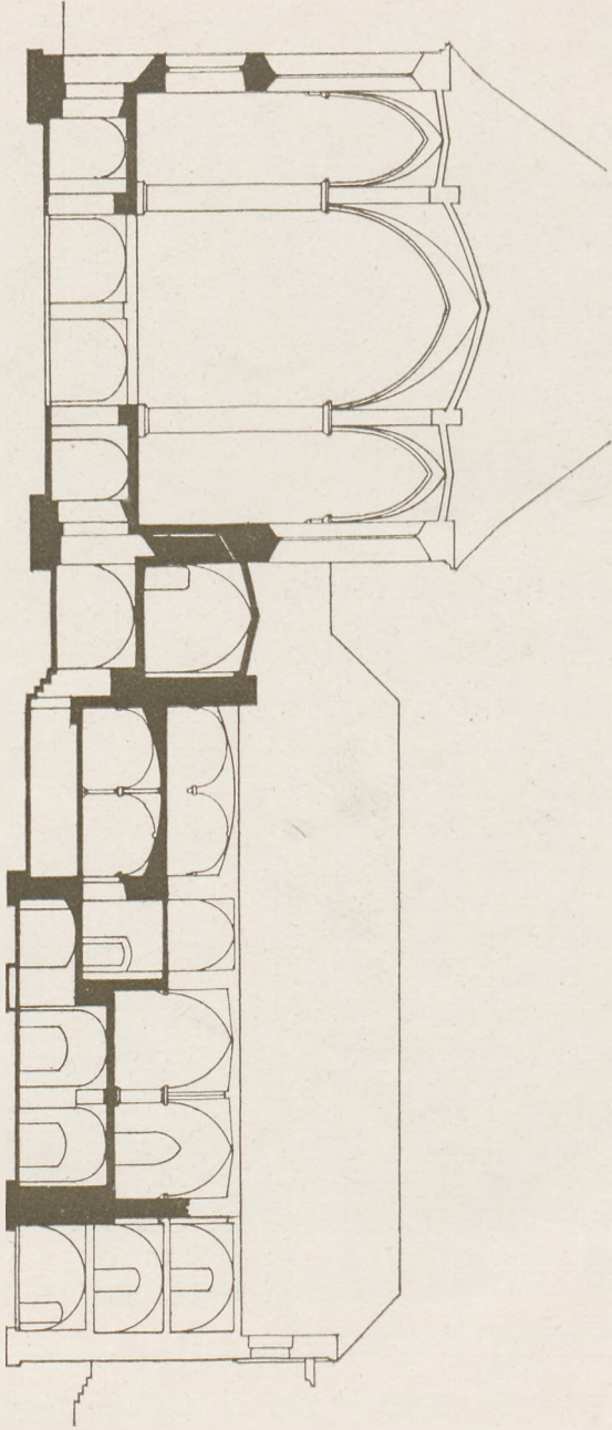
Abb. 12. Schnitt durch den Chor und den östlichen Klostertrakt.
