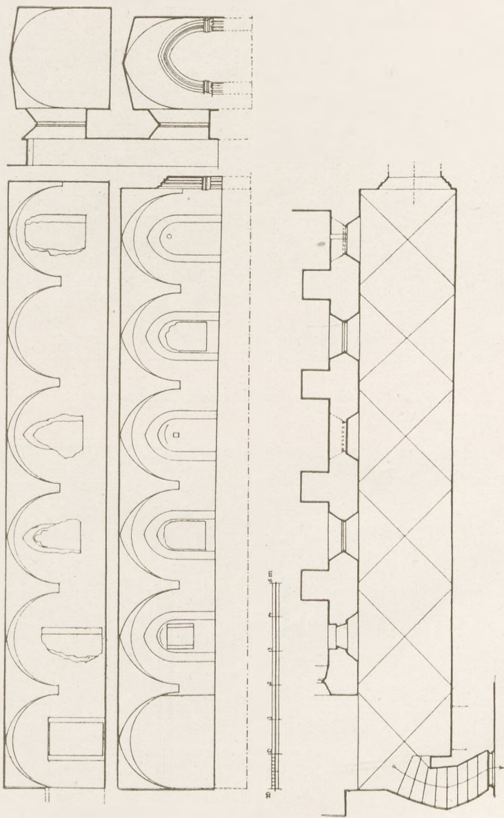
Abb. 20. Grundriss und Schnitt des Ostkreuzganges.
