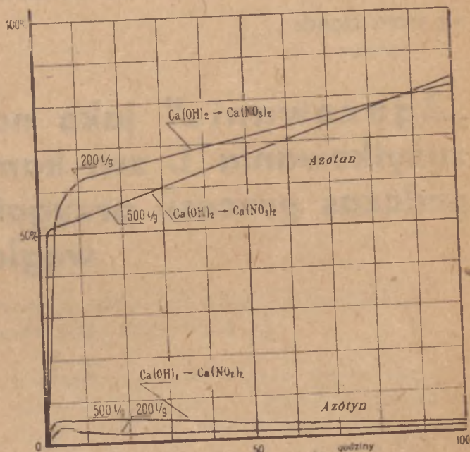
Rus. 8. Wpływ prędkości przepływu gazów nitrujących na przebieg procesu (10 proc. NO 2 ).
