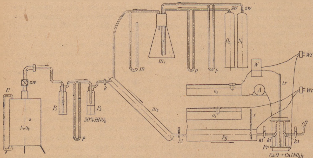
Rys. 1. Schemat aparatury laboratoryjnej do otrzymywania saletry wapniowej.
