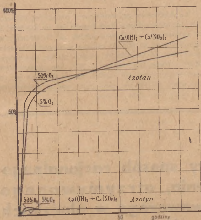
Rus. 7. Wpływ stężenia tlenu w gazach nitrujących na przebieg procesu (10 proc. NO 2 ).
