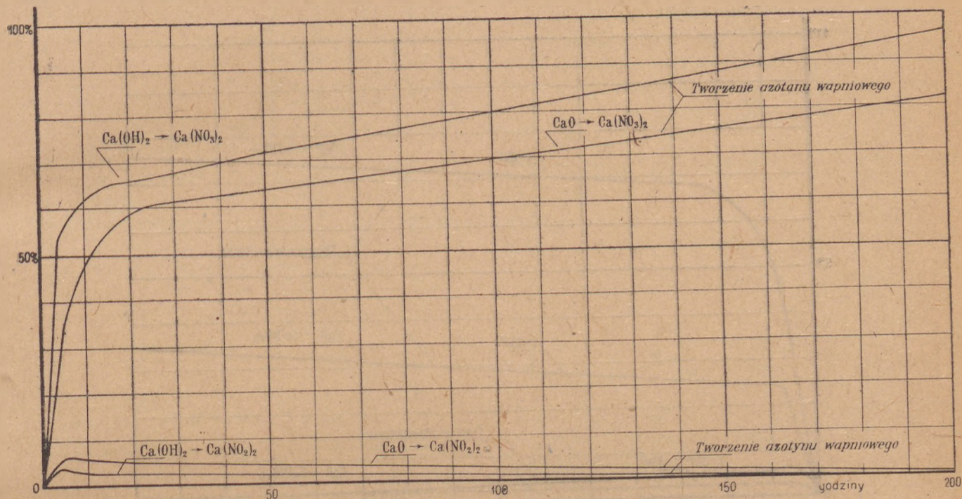
Rys. 2. Wpływ rodzaju materiału nitrowanego na przebieg procesu (10 proc. NO 2 ).
