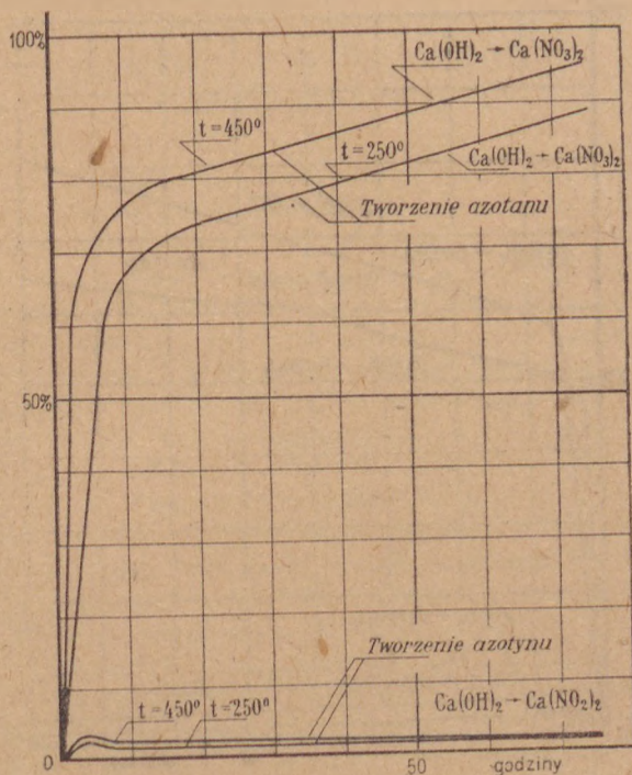
Rys. 3. Wpływ temperatury na przebieg procesu nitrowania wodorotlenku wapnia (10 proc. NO 2 )
