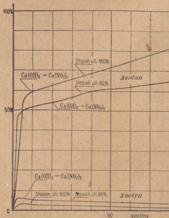
Rys. 6. Wpływ stopnia utlenienia tlenków azotu w gazach nitrujących na przebieg procesu (10 proc. NO 2 ).
