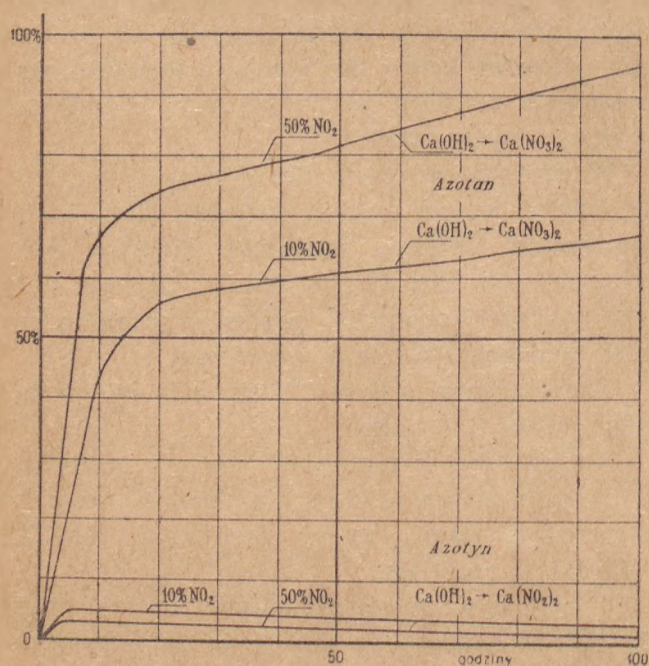
Rys. 5. Wpływ stężenia tlenków azotu w gazach nitrujących na przebieg procesu.
