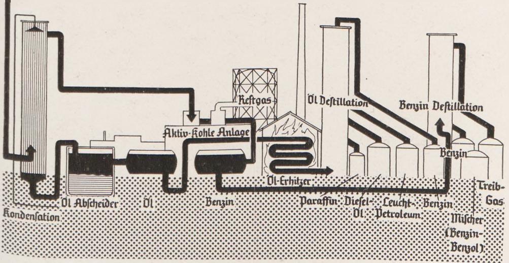
Schema der Herstellung von Benzin aus Kohle
