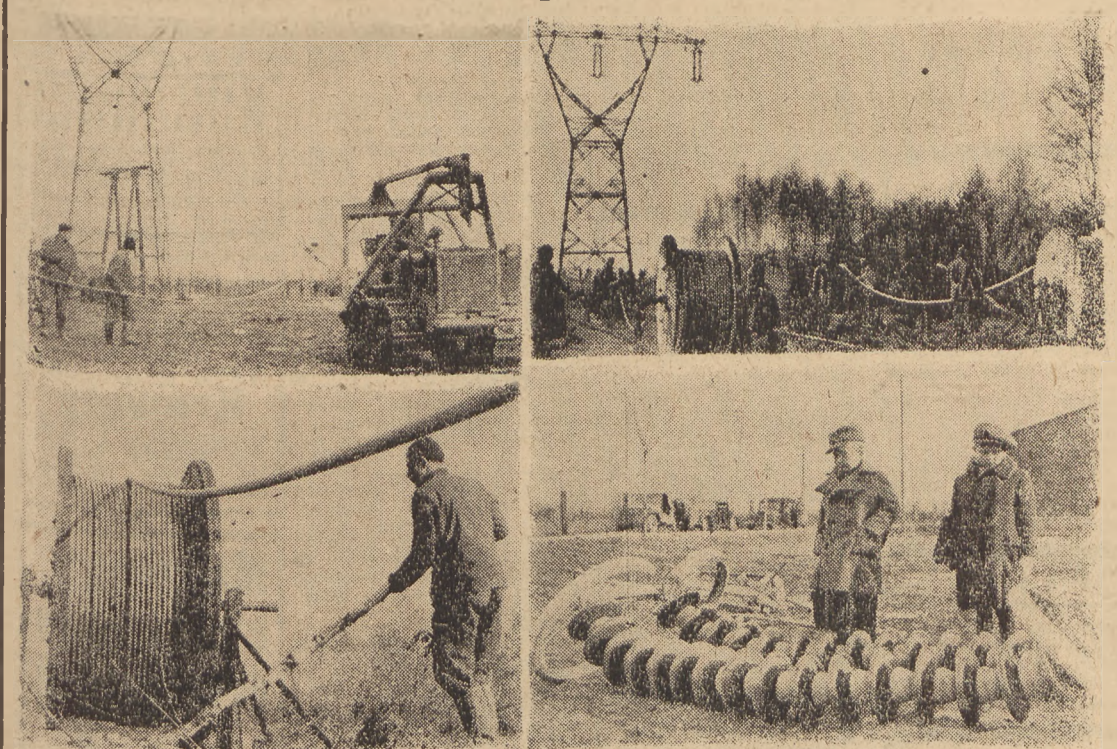
Prace przy linii wysokiego napięcia Łódź - Śląsk dobiegają już końca. Wielki ciągnik wzieje ostatni kabel, który połączy dwie ostatnie wieże. Z prawej: Ogólny widok prac przy zakładaniu kabla. U dołu: Kabel wolno rozwija się ze szpuli. W wypadku zbyt szybkiego rozwijania się robotnik hamuje szpulę. O rozmiarze olbrzymich izolatorów najlepiej świadczy zdjęcie z prawej. Każdy izolator waży 180 kg. Fot. H. Makarewiczowa
