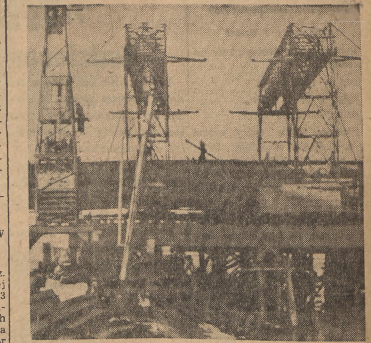
Na moście Śląsko - Dąbrowskim w Warszawie przystąpiono już do montażu jezdnii
