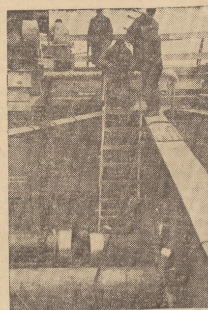
Na całym odcinku trasy „W—Z“ ekipy robotników miejskich Wydziału Wodociągów i Kanalizacji wystąpiły do zakładania przewodów wodociągowych. Na zdjęciu — fragment tych prac.
