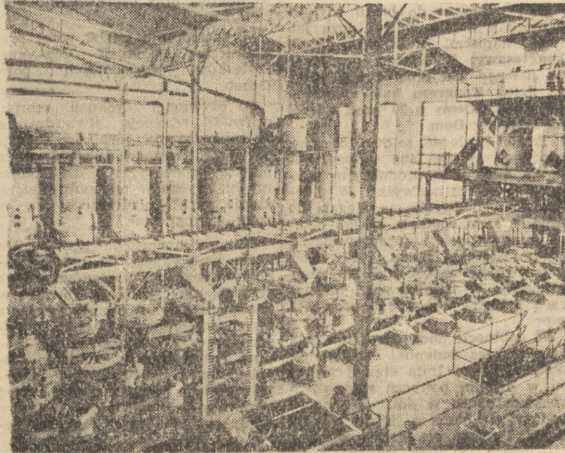
Stacja dyfuzyjna i wyparka
