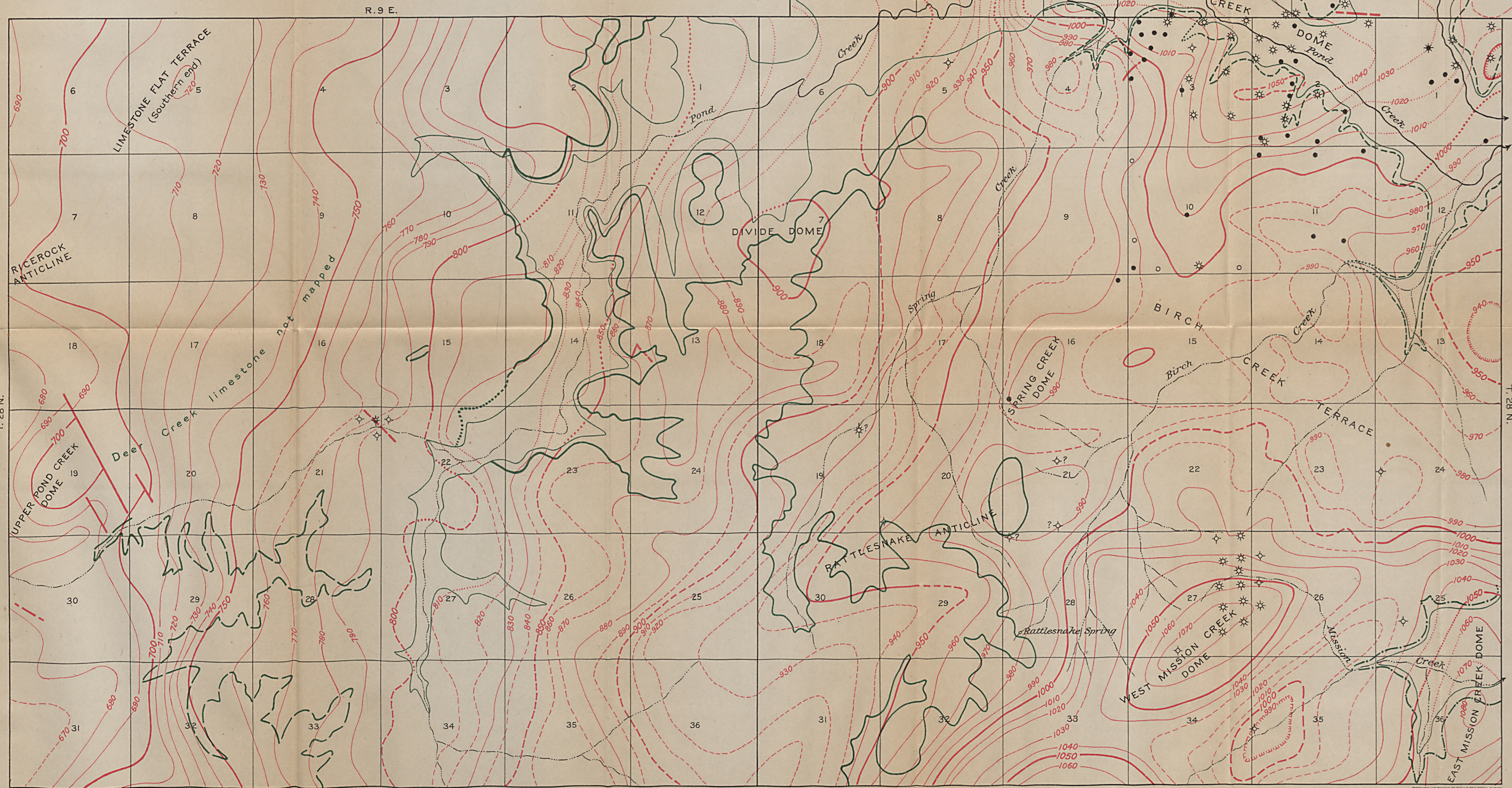
MAP SHOWING GEOLOGIC STRUCTURE OF T. 28 N., R. 9 AND 10 E., AND T. 29 N., R. 10 E.
