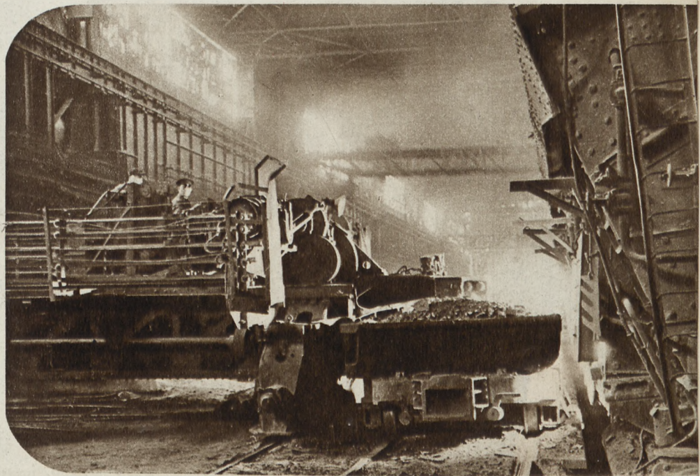
Механическая завалка мартеновской печи на заводе „Азовсталь”.
