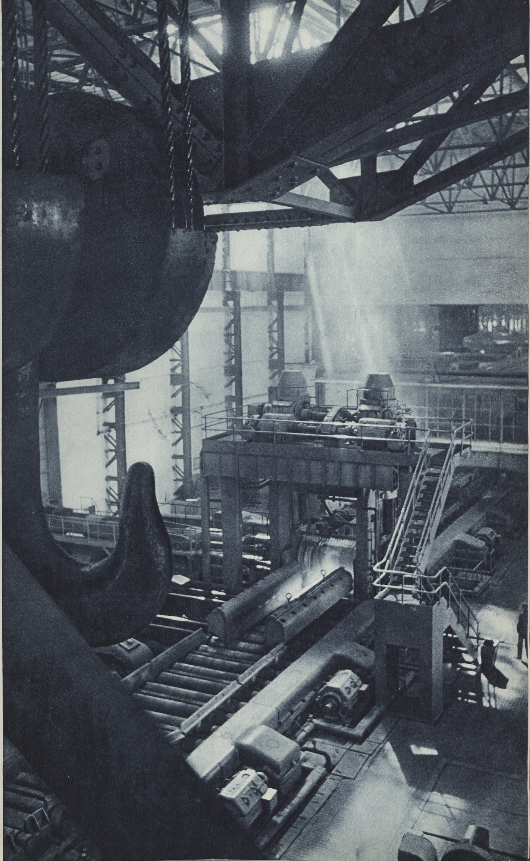
Прокатный цех „Азовстали”. Здесь работает крупнейший в Советском Союзе блюминг.
